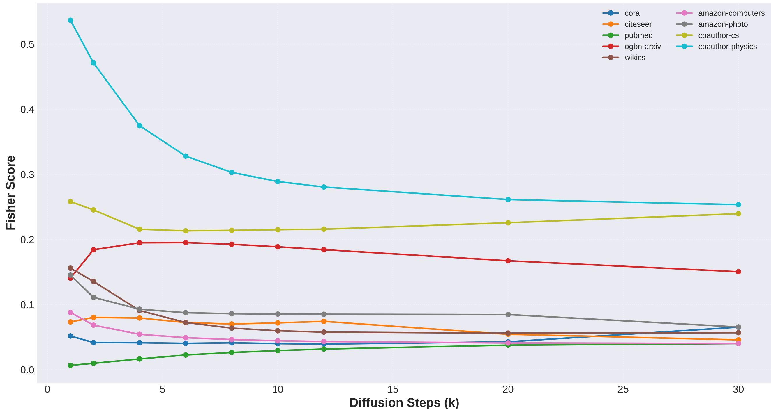
Fisher Score of \|U_i\| vs Diffusion Depth
