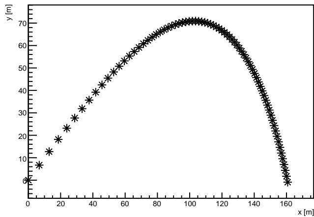
Projectile y vs x
