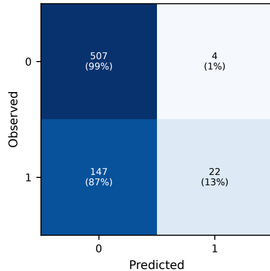
MLP
