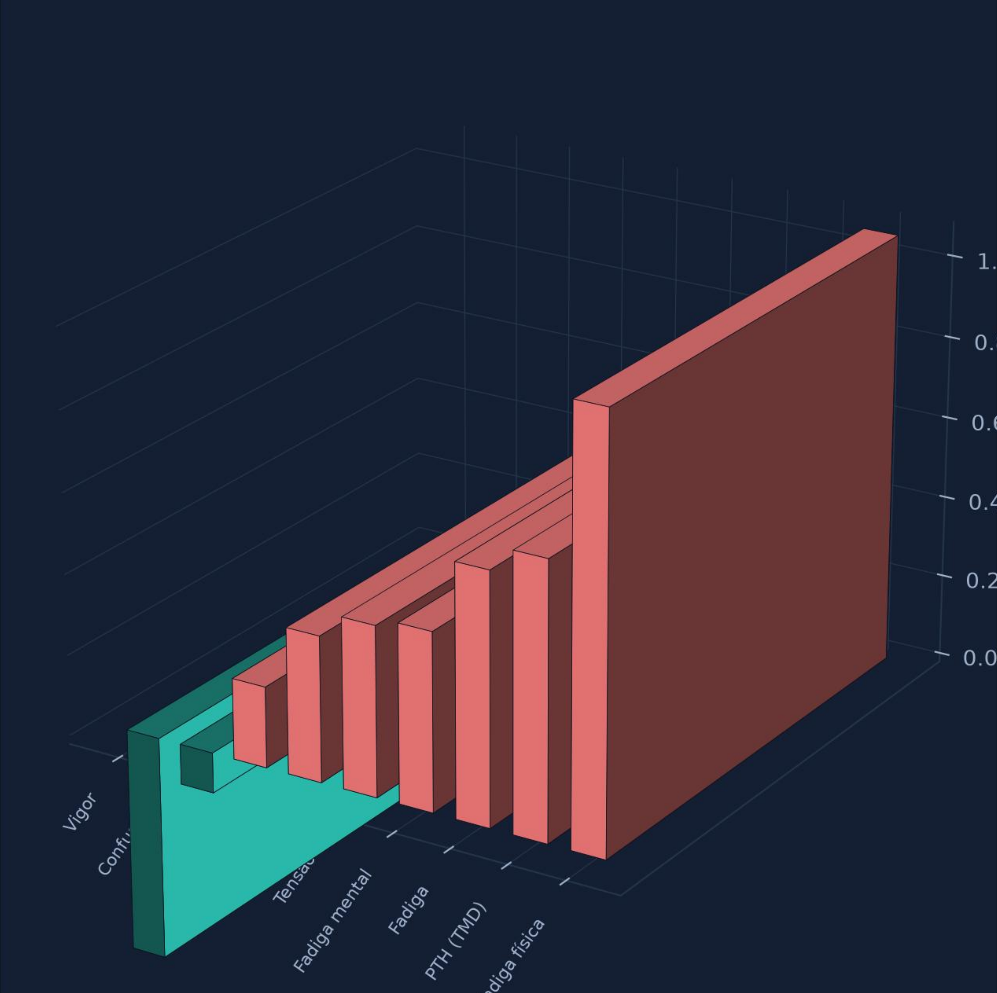
A · Resposta aguda (barras 3D)
