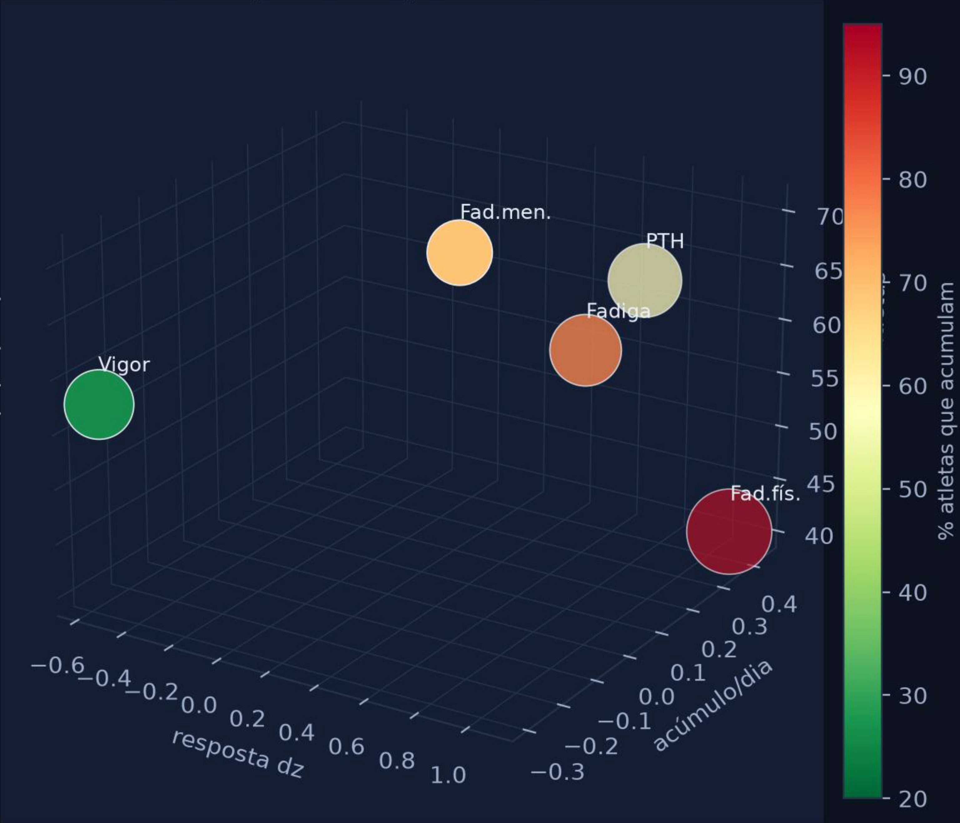
B · Mapa 4D (dispersão 3D + cor)
