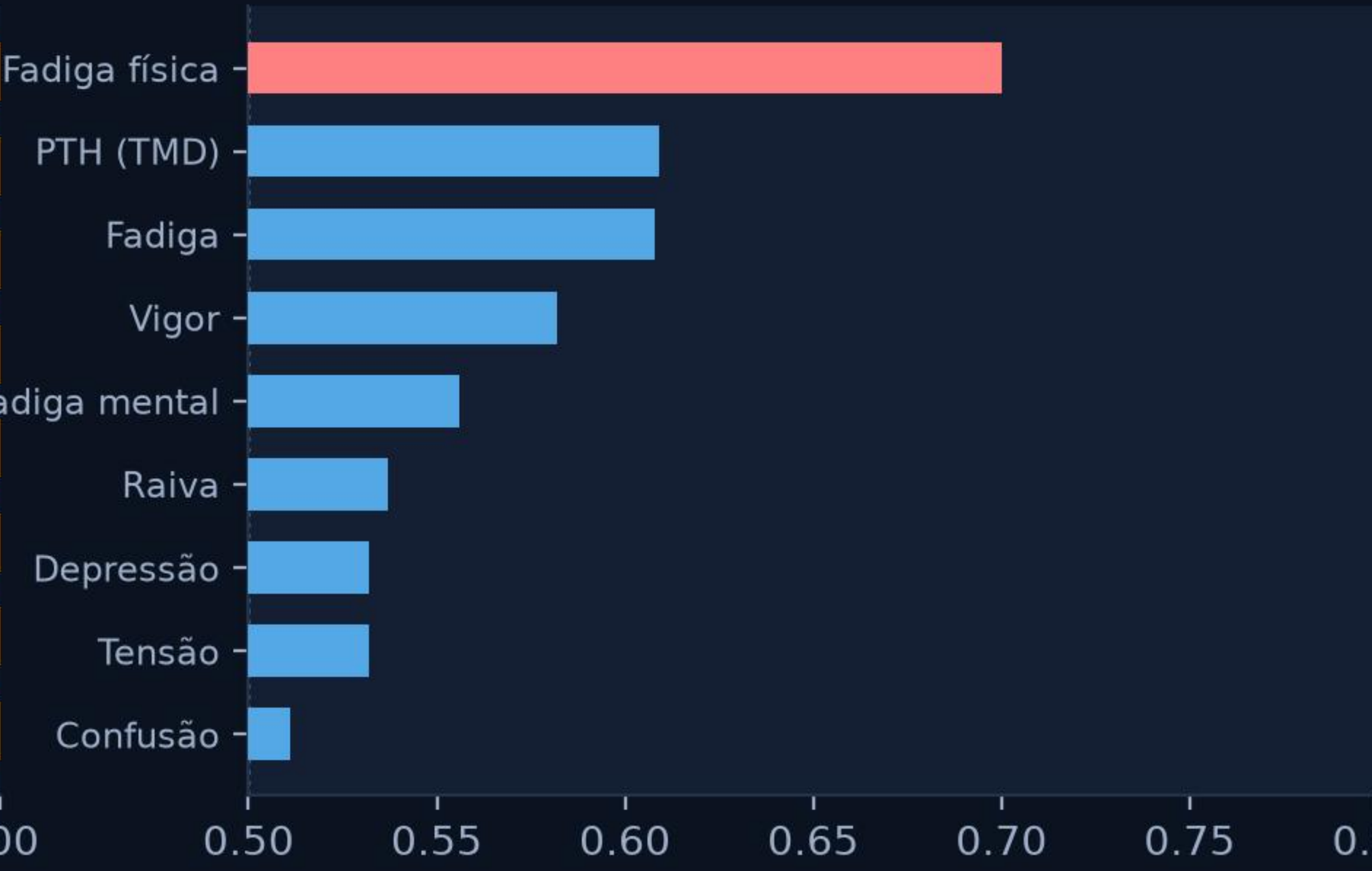
ROC — AUC (separar pós de pré)
