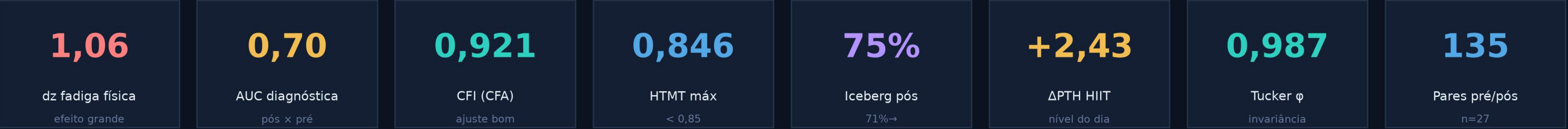
Resposta aguda pré→pós — dz (IC95%)
