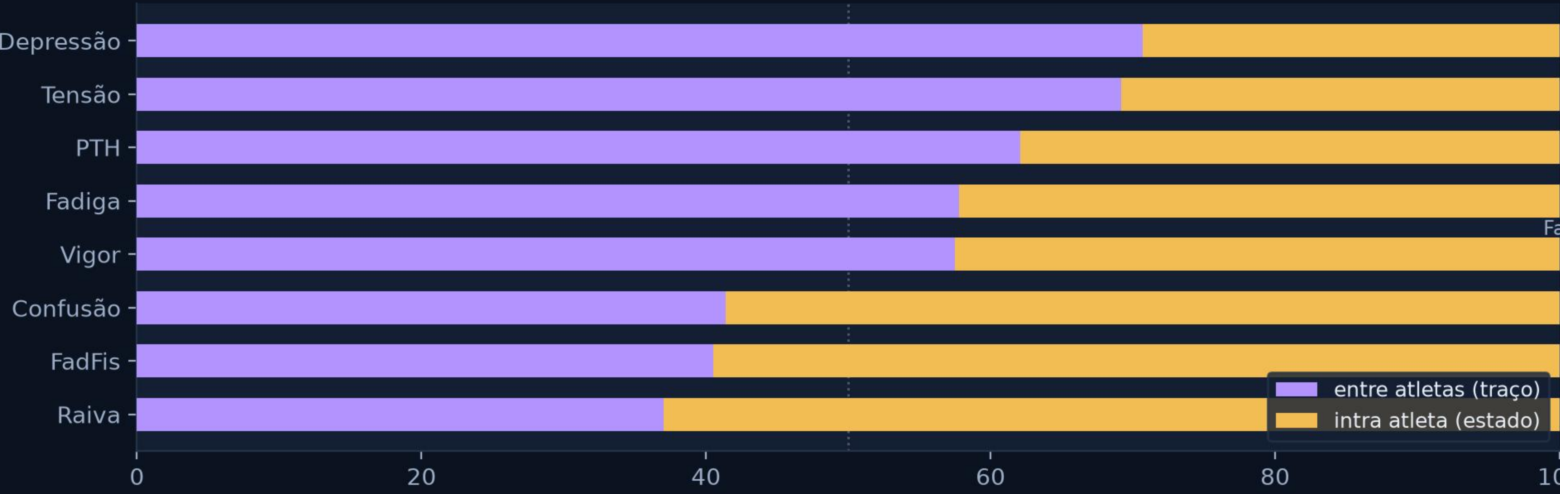
Decomposição da variância (% entre × intra atleta)
