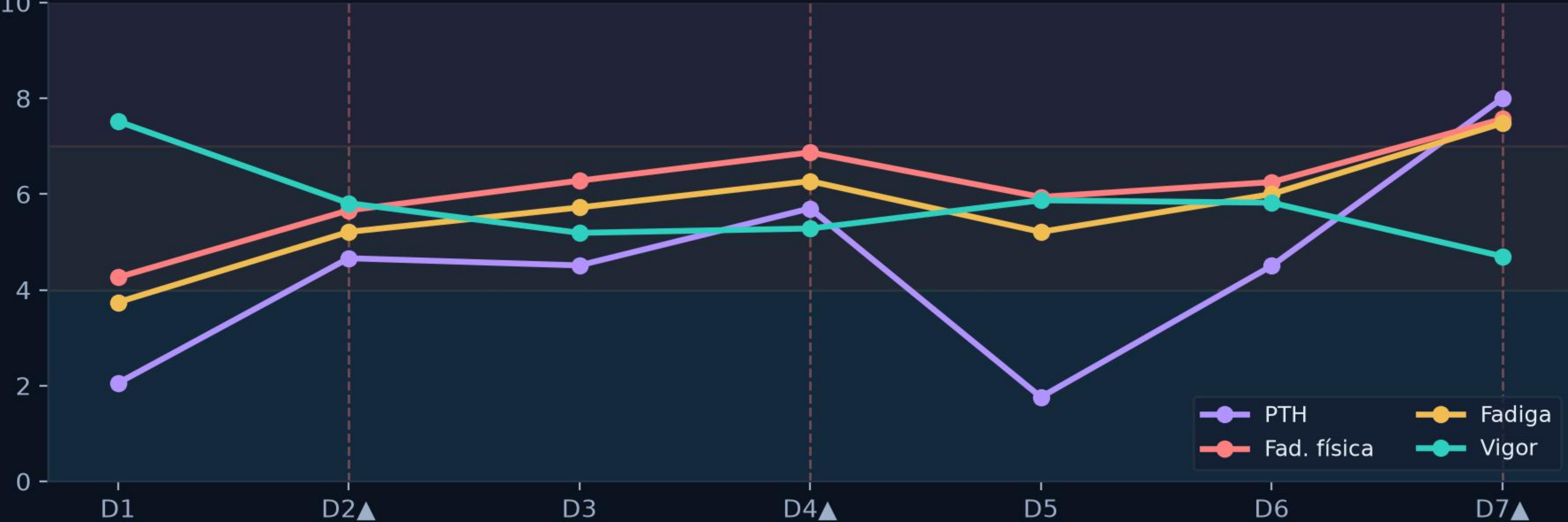
Monitoramento diário da carga de humor (D1→D7)
