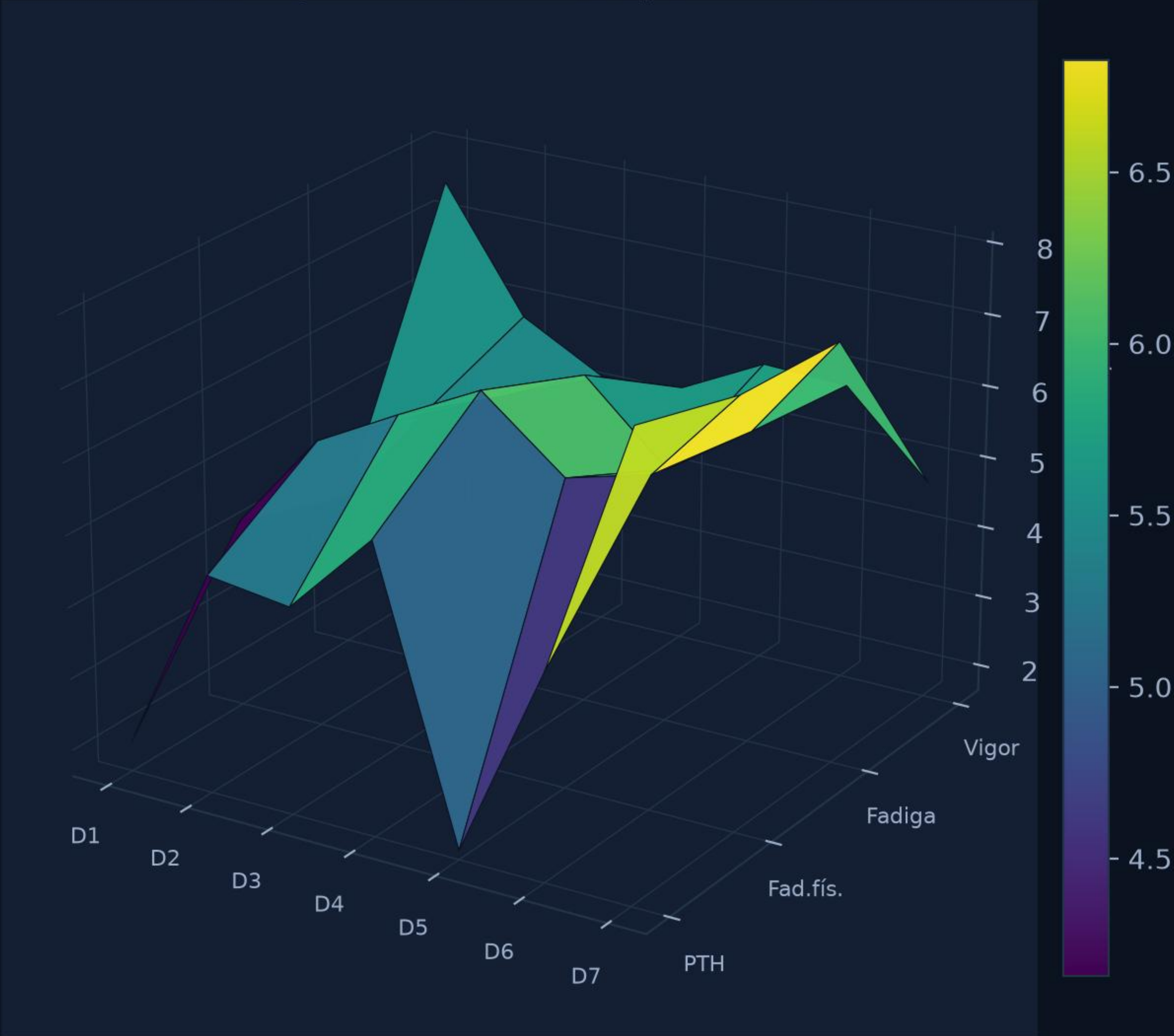
C · Trajetória semanal (superfície 3D)
