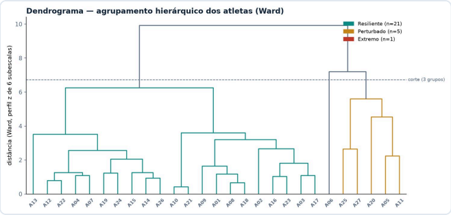
Dendrograma (Ward) dos 27 atletas — corte em 3 grupos.
