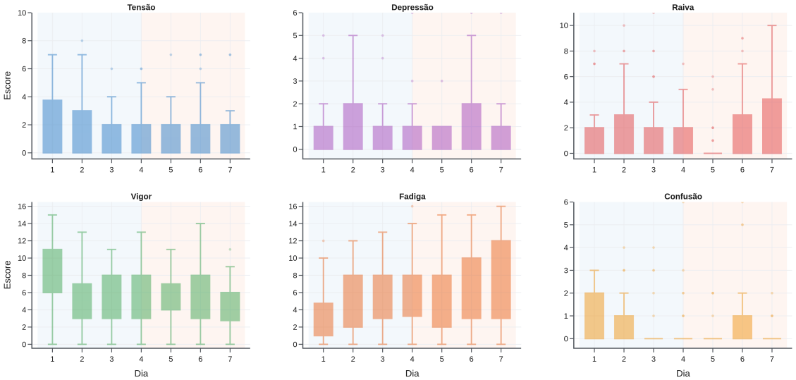
Figura 3 – Diagramas de caixa (box plot) das seis dimensões do BRUMS por dia da semana.
