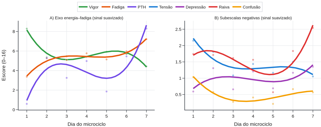
Figura 16 – Trajetórias diárias suavizadas: sinal (curva) sobreposto às médias diárias observadas (pontos), com separação entre a tendência e oruído. A) eixo energia–fadiga; B) subescalas negativas.
