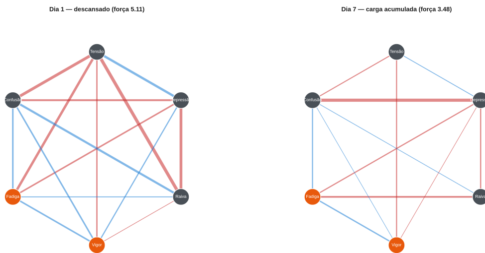
Figura 19 – Redes de correlações parciais (modelo gráfico gaussiano) das seis dimensões do BRUMS no dia descansado (Dia 1) e no dia de maior carga (Dia 7). Arestas vermelhas: associação parcial positiva; azuis: negativa; a espessura é proporcional à magnitude. Vigor e fadiga destacados em laranja.
