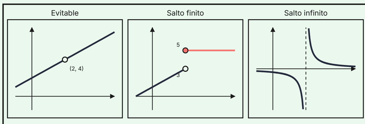
Figura 1: En x = 2 : discontinuidad evitable (hueco en una recta), de salto finito (la función salta de 3 a 5) y de salto infinito (asíntota vertical).
