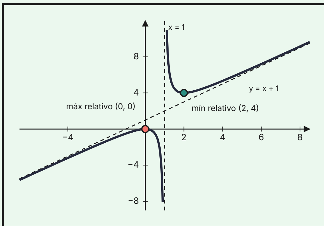
Figura 2: Gráfica de f(x) = \frac{x^2}{x-1} con sus asintotas x = 1 e y = x + 1 , su máximo relativo en el origen y su mínimo relativo en (2, 4) .
