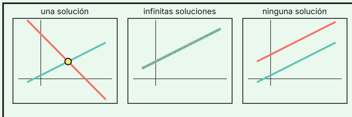
Figura 1: Cada ecuación es una recta: según se corten, coincidan o sean paralelas, el sistema tiene una, infinitas o ninguna solución.
