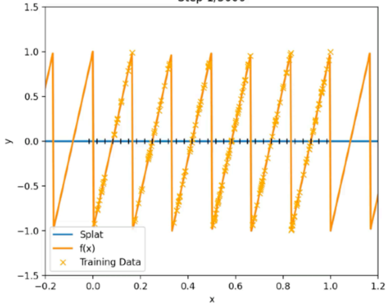
Step 1/3000
