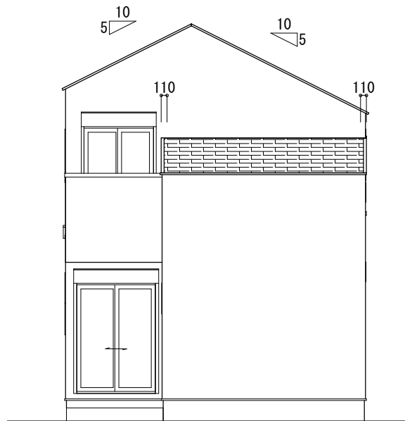
南東立面図 S = 1 / 100
