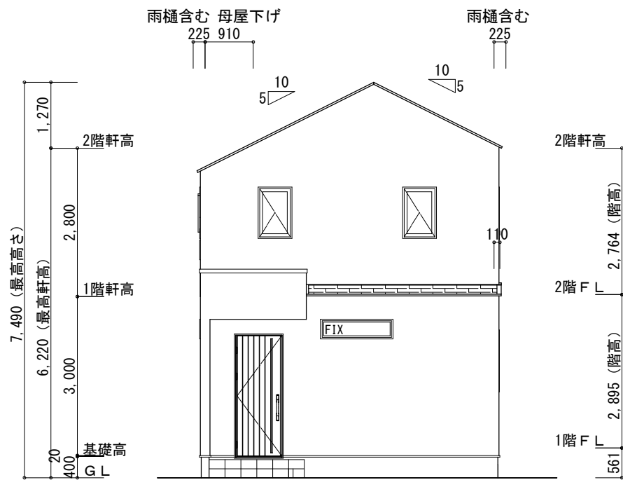
北西立面図 S = 1 / 100
