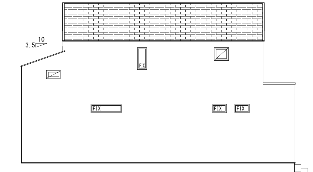
北東立面図 S = 1 / 100
