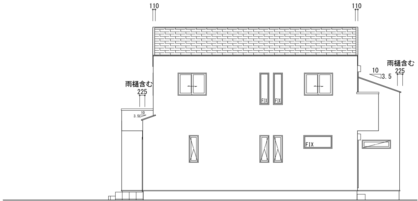
南西立面図 S = 1 / 100
