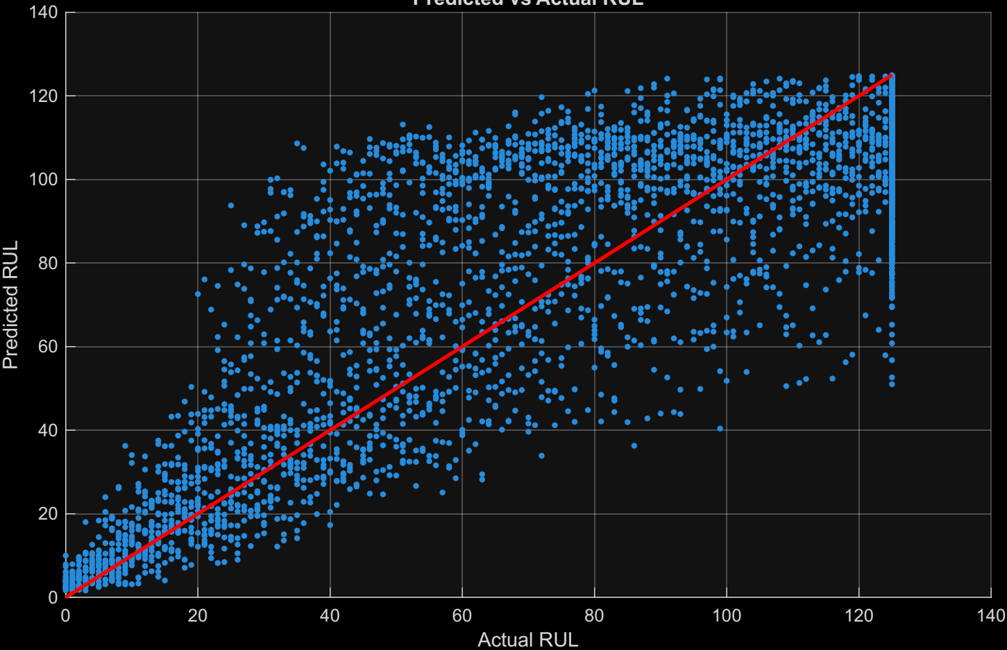
Predicted vs Actual RUL
