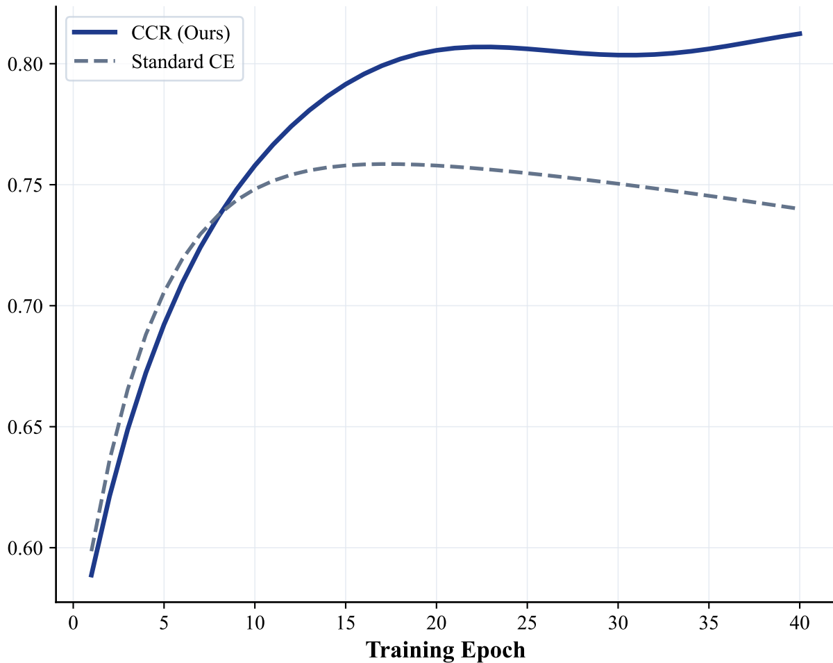
Validation Macro-F1
