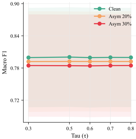
Macro F1 vs \tau
