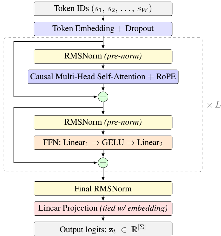
Hình 3.4: Sơ đồ kiến trúc mô hình Transformer Teacher (Decoder-only).
