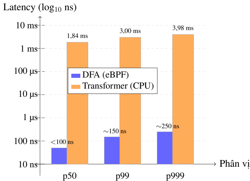
Hình 5.12: So sánh latency DFA (eBPF) và Transformer (CPU) tại p50, p99 và p999 trên thang log 10 . Giá trị DFA là trung điểm của bucket tương ứng trong histogram E1. DFA thấp hơn Transformer hơn 4 bậc độ lớn ở mọi phân vị.
