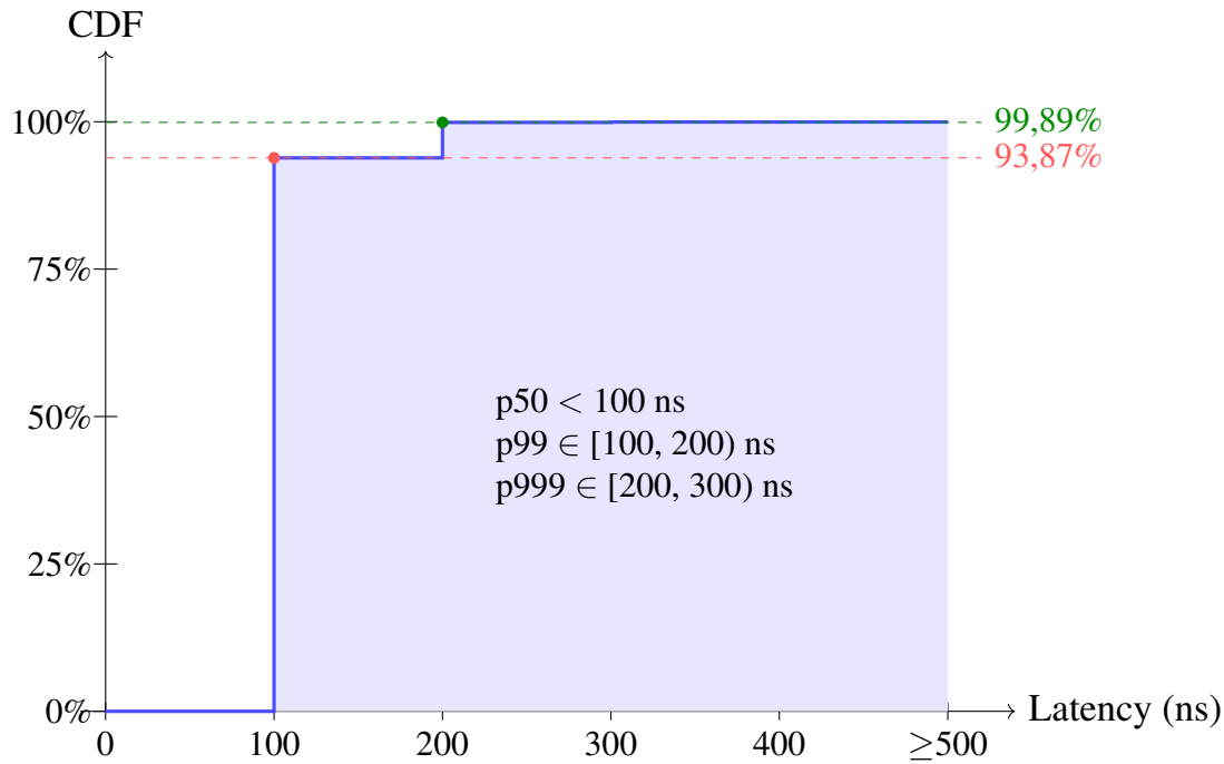
Hình 5.10: CDF latency eBPF DFA trong điều kiện E3 embedded (34.550.232 samples, nginx worker only). Mỗi bước trên trục x tương ứng một bucket 100 ns. CDF nhảy từ 0% lên 93,87% ngay tại mốc 100 ns, cho thấy hơn 9 trong 10 syscall hoàn thành DFA lookup trong dưới 100 ns.
