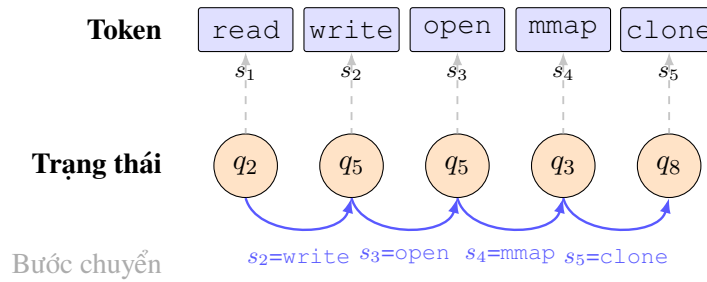
Hình 3.6: Ví dụ xây dựng quan hệ chuyển đổi từ một đoạn chuỗi token. K-Means gán mỗi vector trạng thái ẩn h_t vào một cụm (hàng giữa). Mỗi cặp liên tiếp (q_i, s_{t+1}) \rightarrow q_j đóng góp một ứng viên vào bảng chuyển trạng thái thô (hàng dưới). Hai bước chuyển liên tiếp (q_2, write) \rightarrow q_5 và (q_5, open) \rightarrow q_5 minh họa trường hợp một trạng thái tự lặp sau khi nhận token đầu vào mới.
