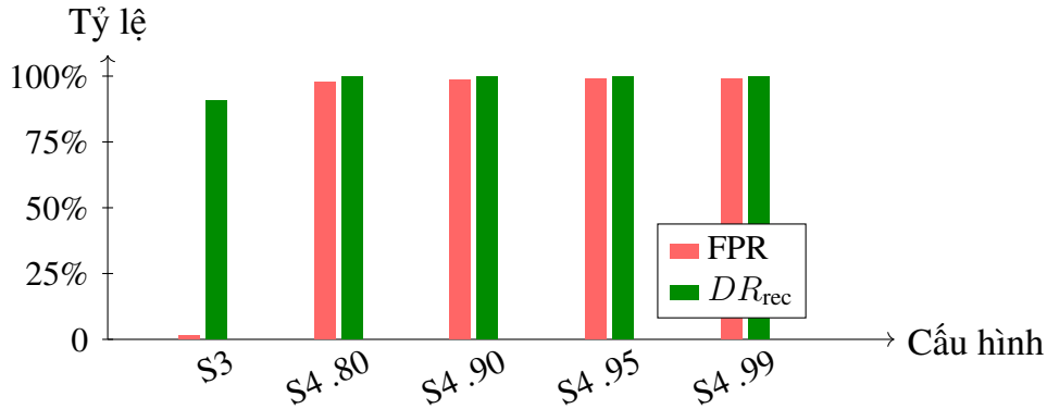
Hình 5.7: Đánh đổi giữa FPR và DR_{rec} của các chiến lược DFA. S1 không xuất hiện vì gặp bùng nổ trạng thái và không tạo được DFA hoàn chỉnh. S4 đạt DR_{rec} tuyệt đối bằng cách gán attack cho gần như toàn bộ window normal, nên không thể dùng trong triển khai.
