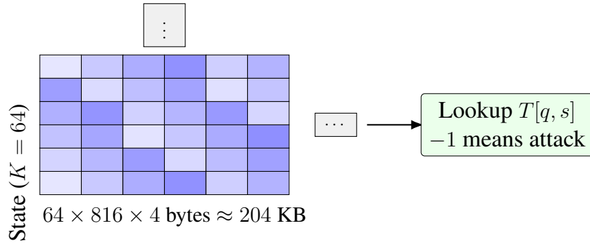
Hình 5.9: Biểu diễn bảng chuyển DFA dưới dạng mảng trực tiếp. Kích thước của cấu hình S3 đủ nhỏ để nạp vào BPF map và cho phép tra cứu trạng thái kế tiếp bằng một phép chỉ mục hóa hằng số.
