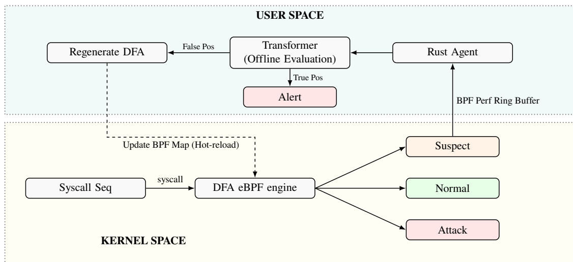
Hình 3.2: Cơ chế tương tác động và vòng lặp cập nhật giữa Kernel-space và User-space
