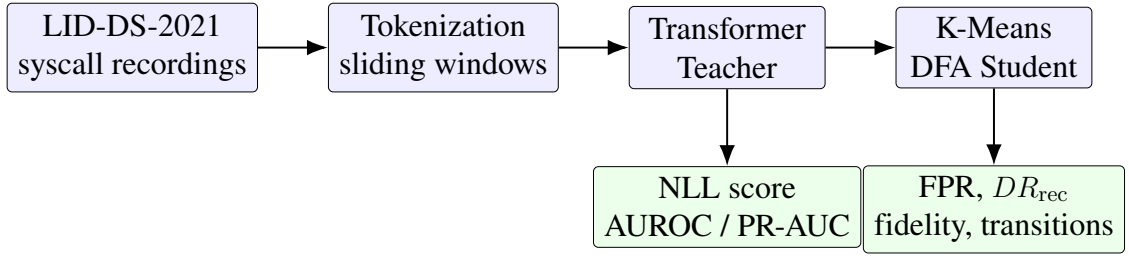
Figure 5.1: Pipeline đánh giá thực nghiệm. Transformer Teacher tạo điểm bất thường liên tục bằng NLL, trong khi DFA Student thay điểm số liên tục bằng kiểm tra bước chuyển trạng thái đã từng xuất hiện trong dữ liệu huấn luyện bình thường.
