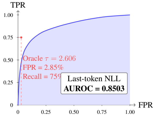
Figure 5.3: Đường cong ROC của điểm last-token NLL ở cấp độ window. Diện tích dưới đường cong đạt 0.8503, cho thấy Teacher xếp hạng window attack cao hơn window normal trong phần lớn các cặp so sánh, dù nhãn attack của LID-DS có nhiều cấu trúc.
