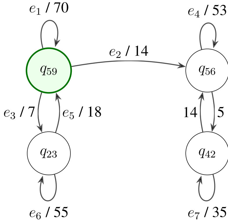
Figure 5.8: Một graph con được lấy trực tiếp từ bảng chuyển DFA S3 tại K = 64 . Mỗi cạnh gom các dòng có cùng cặp state nguồn–đích; nhãn trên cạnh có dạng mã cạnh / số syscall token. Start state của bảng chuyển là q_{59} và toàn bộ DFA S3 có 1,973 transitions.
