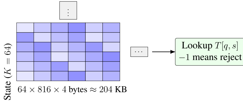
Figure 5.9: Biểu diễn bảng chuyển DFA dưới dạng mảng trực tiếp. Kích thước của cấu hình S3 đủ nhỏ để nạp vào BPF map và cho phép tra cứu trạng thái kế tiếp bằng một phép chỉ mục hóa hằng số.
