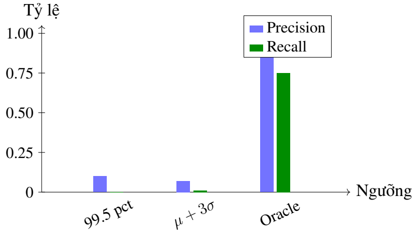
Figure 5.4: So sánh precision và recall attack tại ba cách chọn ngưỡng. Ngưỡng oracle thể hiện năng lực tiềm năng của điểm NLL, nhưng không phải ngưỡng vận hành vì cần nhãn test.
