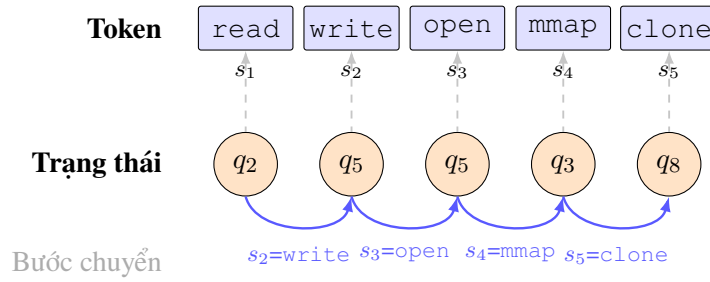
Figure 3.4: Ví dụ xây dựng quan hệ chuyển đổi từ một đoạn chuỗi token. K-Means gán mỗi vector trạng thái ẩn h_t vào một cụm (hàng giữa). Mỗi cặp liên tiếp (q_i, s_{t+1}) \rightarrow q_j đóng góp một ứng viên vào bảng chuyển trạng thái thô (hàng dưới). Hai bước chuyển liên tiếp (q_2, \text{write}) \rightarrow q_5 và (q_5, \text{open}) \rightarrow q_5 minh họa trường hợp một trạng thái tự lặp sau khi nhận token đầu vào mới.
