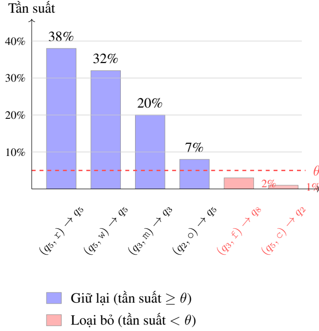
Figure 3.5: Minh họa chiến lược S4 Statistical Pruning. Các bước chuyển (ví dụ minh họa; tên rút gọn: r=read, w=write, m=mmap, o=open, f=futex, c=clone ) được sắp xếp giảm dần theo tần suất. Đường ngưỡng \theta loại bỏ các nhánh thiếu số (màu đỏ), vốn là tạo vật của lượng tử hóa K-Means thay vì hành vi thực sự. Phân phối lệch nặng về nhóm bước chuyển chính là đặc trưng điển hình của workload máy chủ lặp lại cao.
