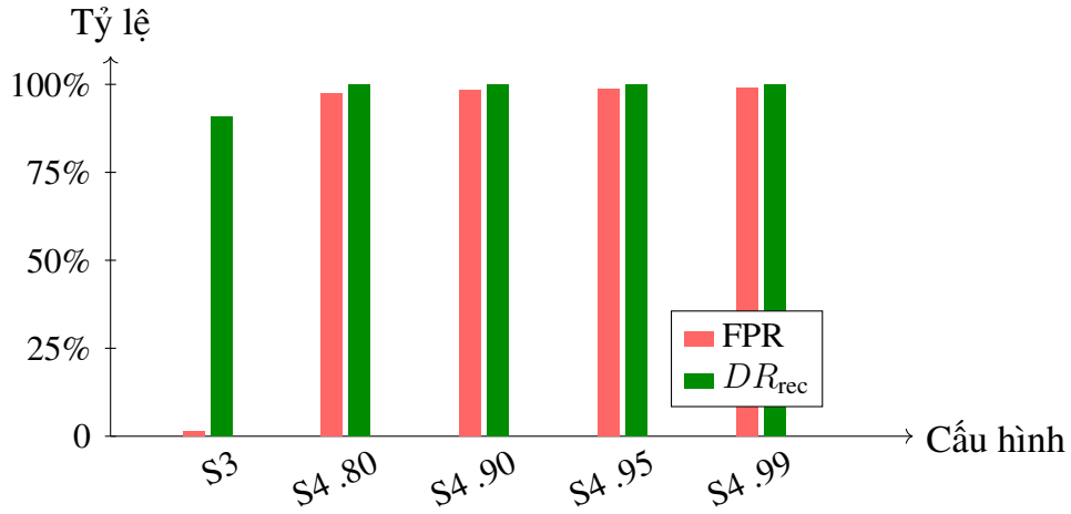
Figure 5.7: Đánh đổi giữa FPR và DR_{rec} của các chiến lược DFA. S4 đạt DR_{rec} tuyệt đối bằng cách từ chối gần như toàn bộ window normal, nên không thể dùng trong triển khai.
