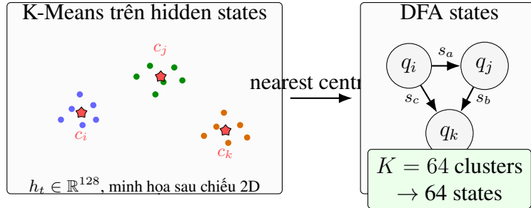
Figure 5.6: Minh họa bước K-Means trong Giai đoạn 3. Các vector hidden state của Teacher được gom quanh các centroid, sau đó mỗi centroid được xem như một trạng thái rời rạc của DFA. Bảng chuyển \delta(q, s) được xây dựng bằng cách quan sát các cặp trạng thái liên tiếp trong chuỗi syscall bình thường.
