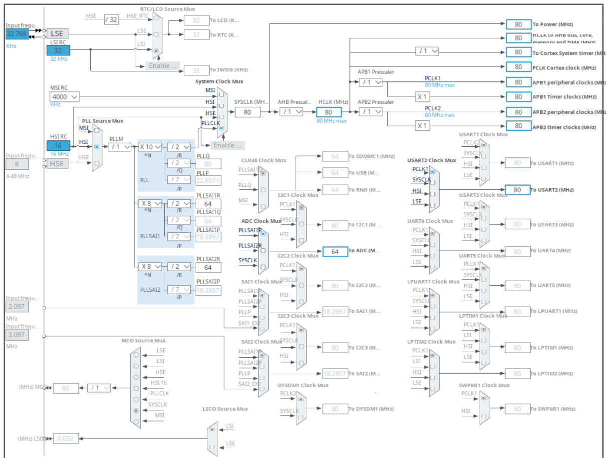
Rysunek 3: Konfiguracja zegarów mikrokontrolera
