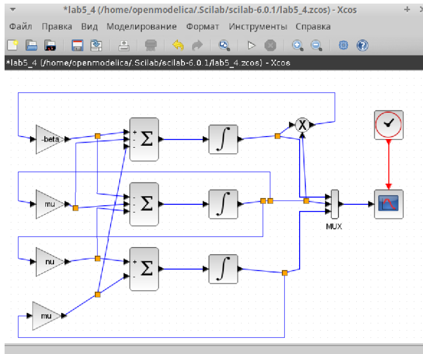
Figure 3.13: Модель SIR с учетом демографических процессов в xcos
