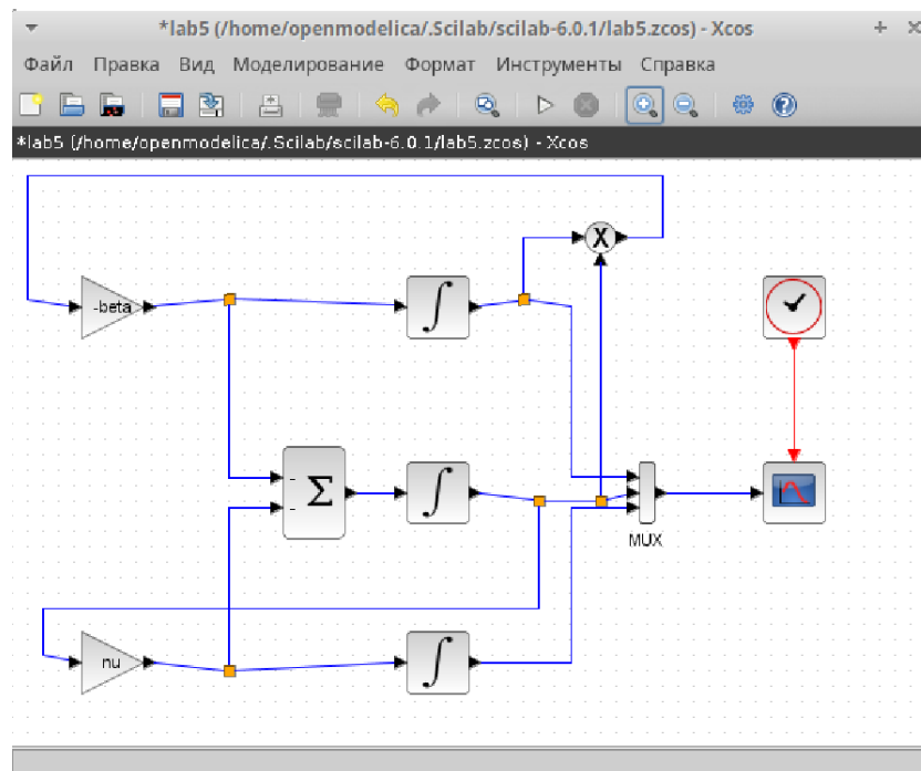
Figure 3.2: Модель SIR в xcos
