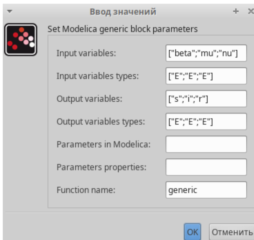
Figure 3.16: Параметры блока Modelica для модели SIR с учетом демографических процессов
