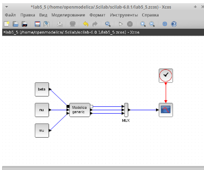
Figure 3.15: Модель SIR с учетом демографических процессов в xcos с применением блока Modelica
