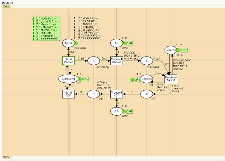
Рис. 5: Модель простого протокола передачи данных
