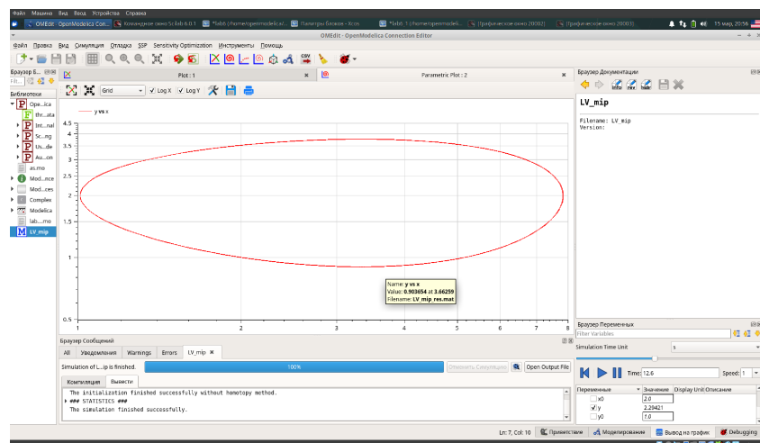
Рис. 3.13: Фазовый портрет модели Лотки-Вольтерры при a = 2, b = 1, c = 0.3, d = 1, x(0) = 2, y(0) = 1
