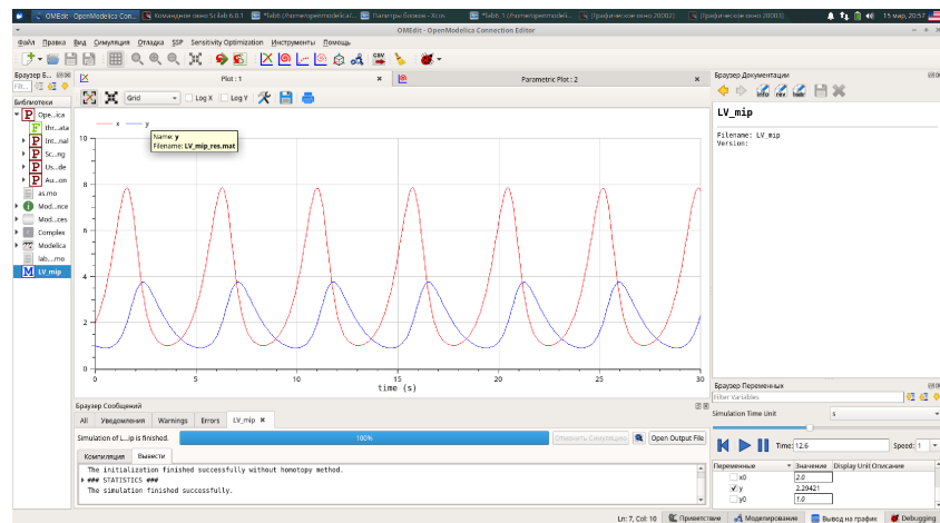
Рис. 3.12: Динамика изменения численности хищников и жертв модели Лотки-Вольтерры при a = 2, b = 1, c = 0.3, d = 1, x(0) = 2, y(0) = 1
