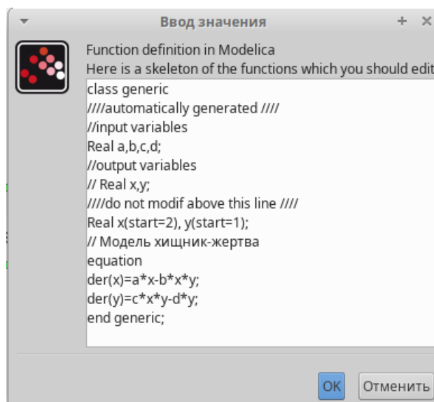
Рис. 3.9: Параметры блока Modelica для модели “хищник-жертва”
