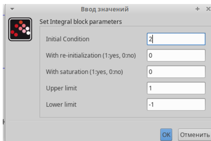
Рис. 3.3: Задание начальных значений в блоках интегрирования
