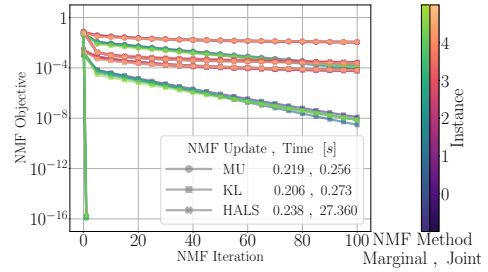
(d) Bond dimension \chi = 16
