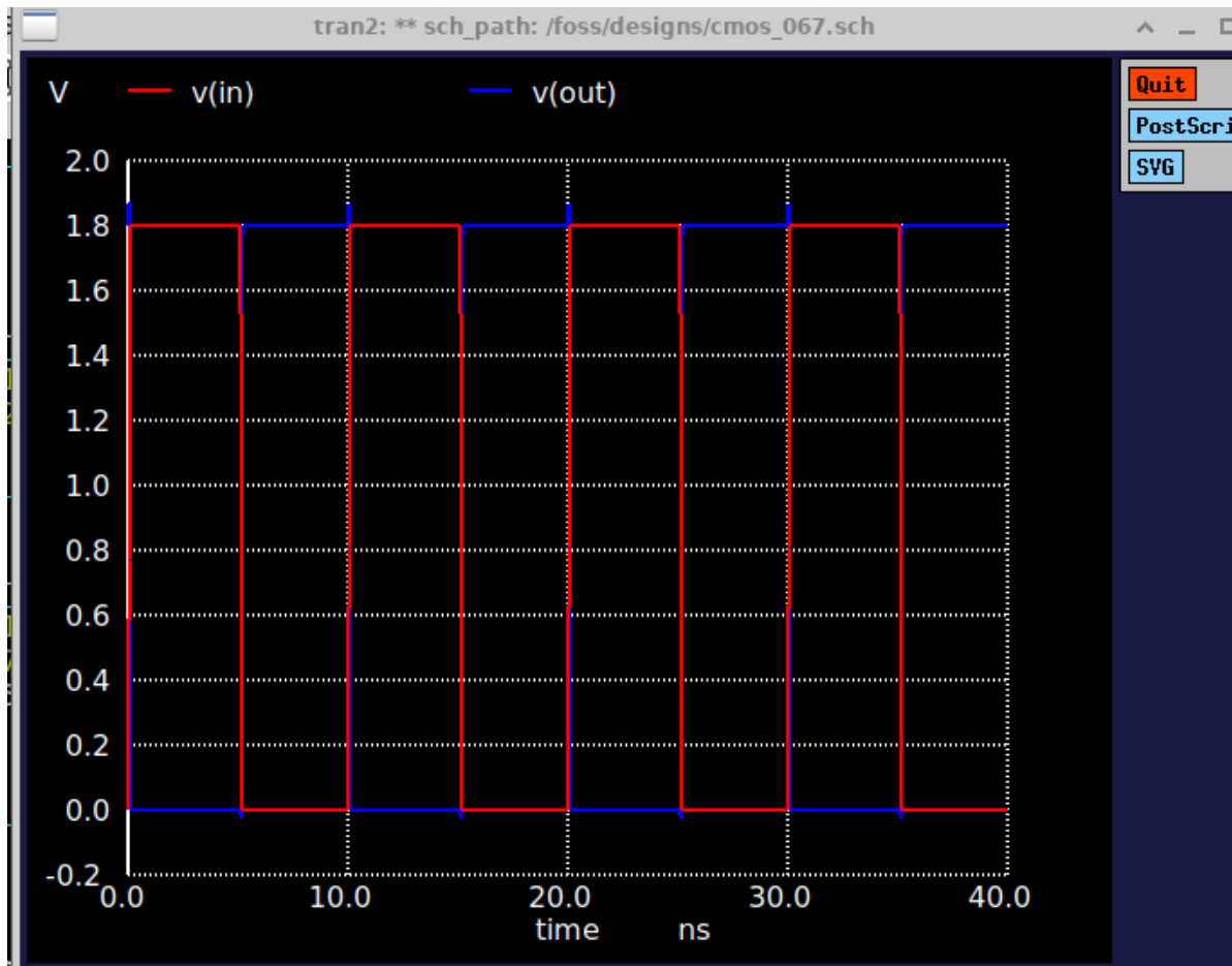
Gambar 2. Hasil simulasi transient V(in) dan V(out)
