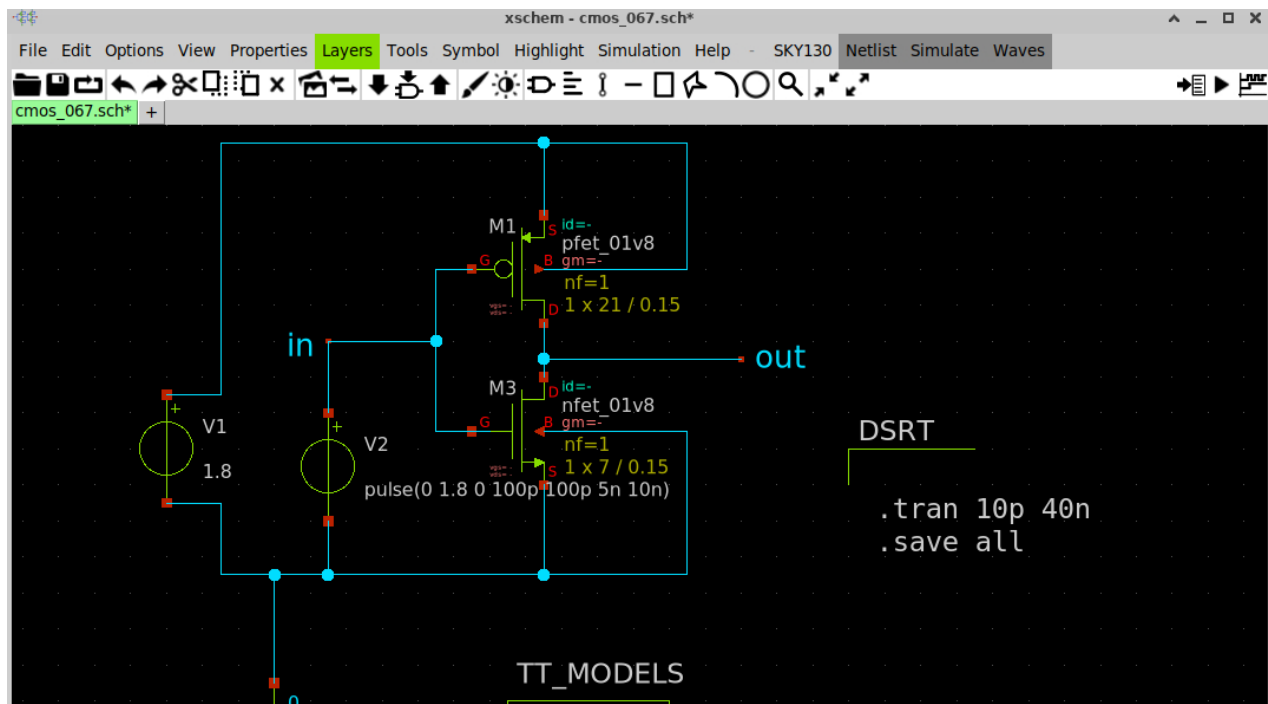
Gambar 1. Schematic CMOS inverter menggunakan Xschem
