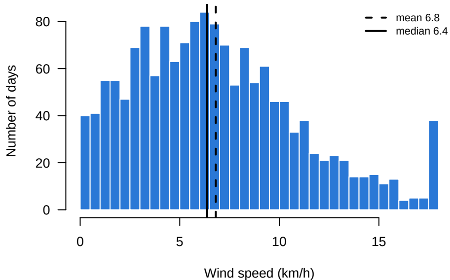
Wind speed (km/h) (skewness 0.62)
