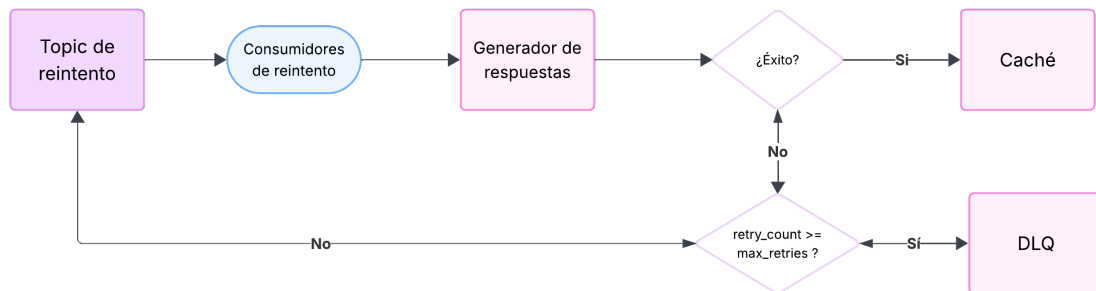
Figura 2: Flujo del sistema para la adición de consultas en la DLQ
