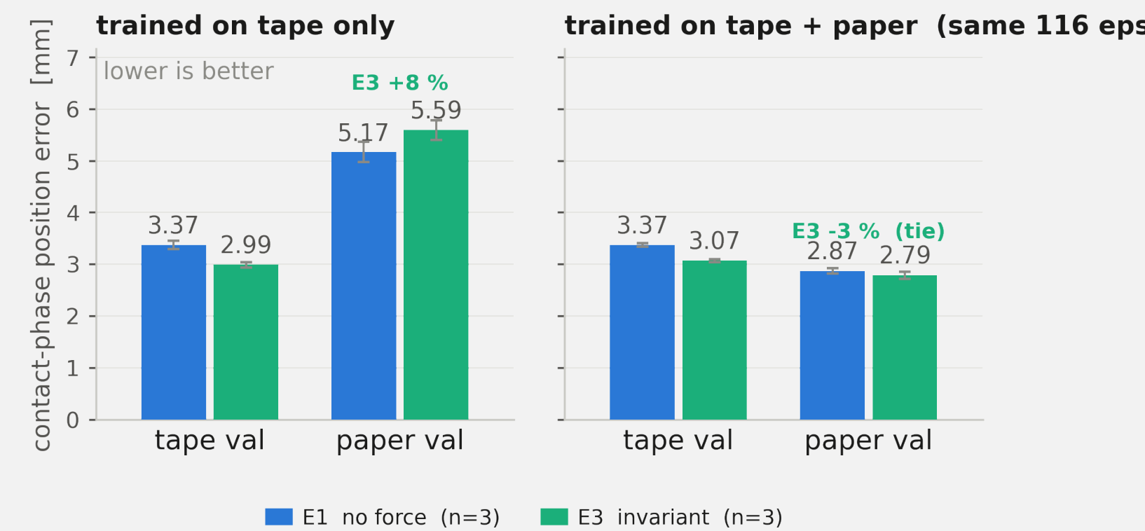
Fig. 5 단일 표면 학습 (왼쪽) 과 혼합 학습 (오른쪽) 에서 E1 vs E3. 종이 값은 검증 34 개 기준이라 표 (150 개 전체) 와 다르다.
