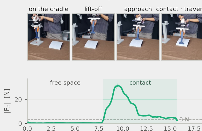
Fig. 3 시연 한 에피소드 — 네 단계와 접촉력 |F|
