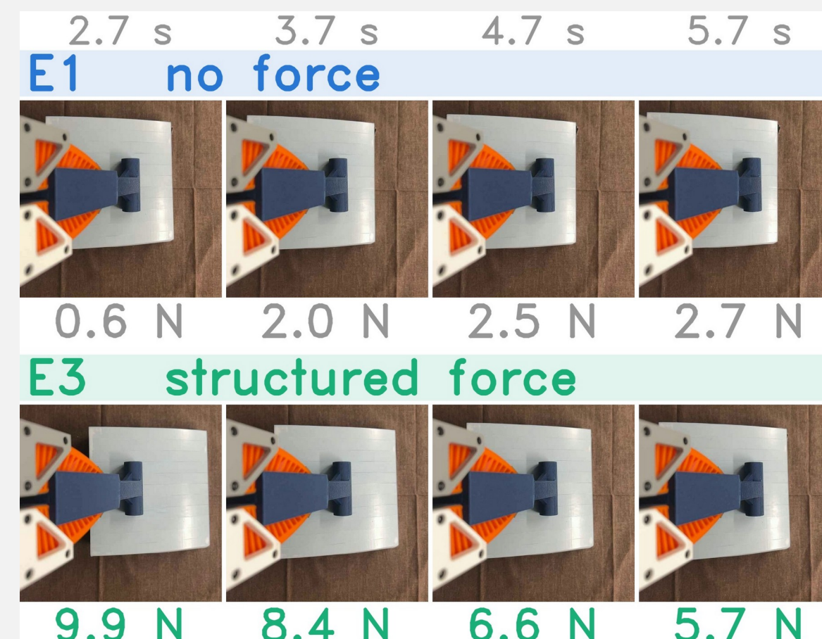
Fig. 8 FR3 페루프 — (왼쪽) 한 회차, 1 초 간격: E1 은 판을 놓친 채 2 N, E3 는 눌러 미끄러진다. (오른쪽) 40 회, 점 = 회차 · 막대 = 평균
