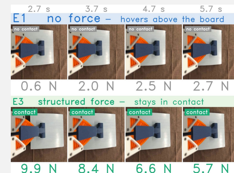
Fig. 7 FR3 페루프 — (왼쪽) 같은 그리퍼 · 물을 단 FR3. (가운데) 한 회차, 1 초 간격. 배지 = 접촉 여부 (|F| ≥ 3 N): E1 은 판 위에 뜬 채 2 N, E3 는 눌러 미끄러진다. (오른쪽) 40 회, 점 = 회차 · 막대 = 평균
