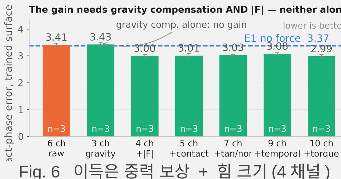
Fig. 6 이득은 중력 보상 + 힘 크기 (4 채널) 에서 나타나고, 그 뒤로는 늘지 않는다
