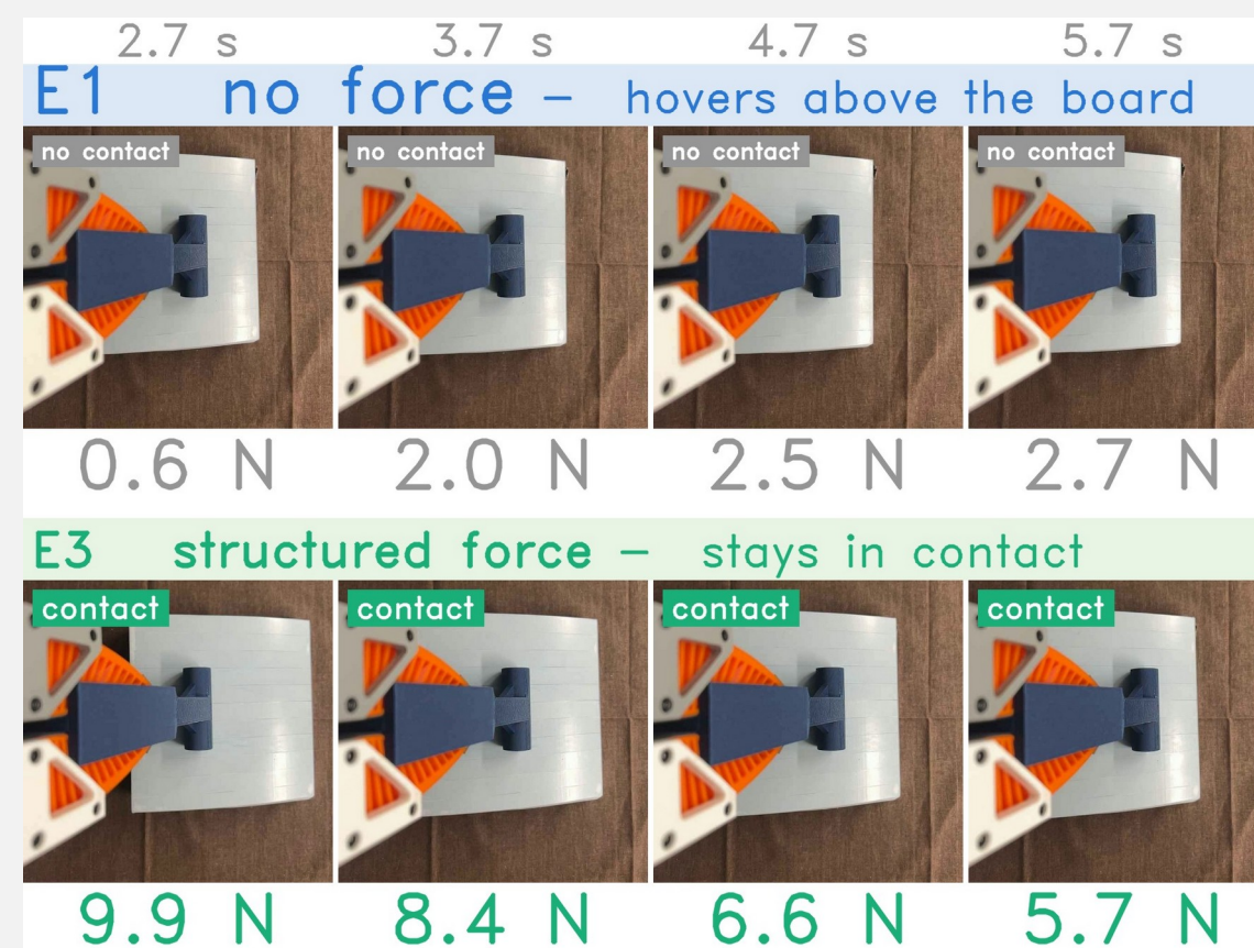
Fig. 8 FR3 페루프 — (왼쪽) 한 회차, 1 초 간격. 배치 = 접촉 여부 ( |F| \geq 3 N): E1 은 판 위에 뜬 채 2 N, E3 는 눌러 미끄러진다. (오른쪽) 40 회, 점 = 회차 · 막대 = 평균
