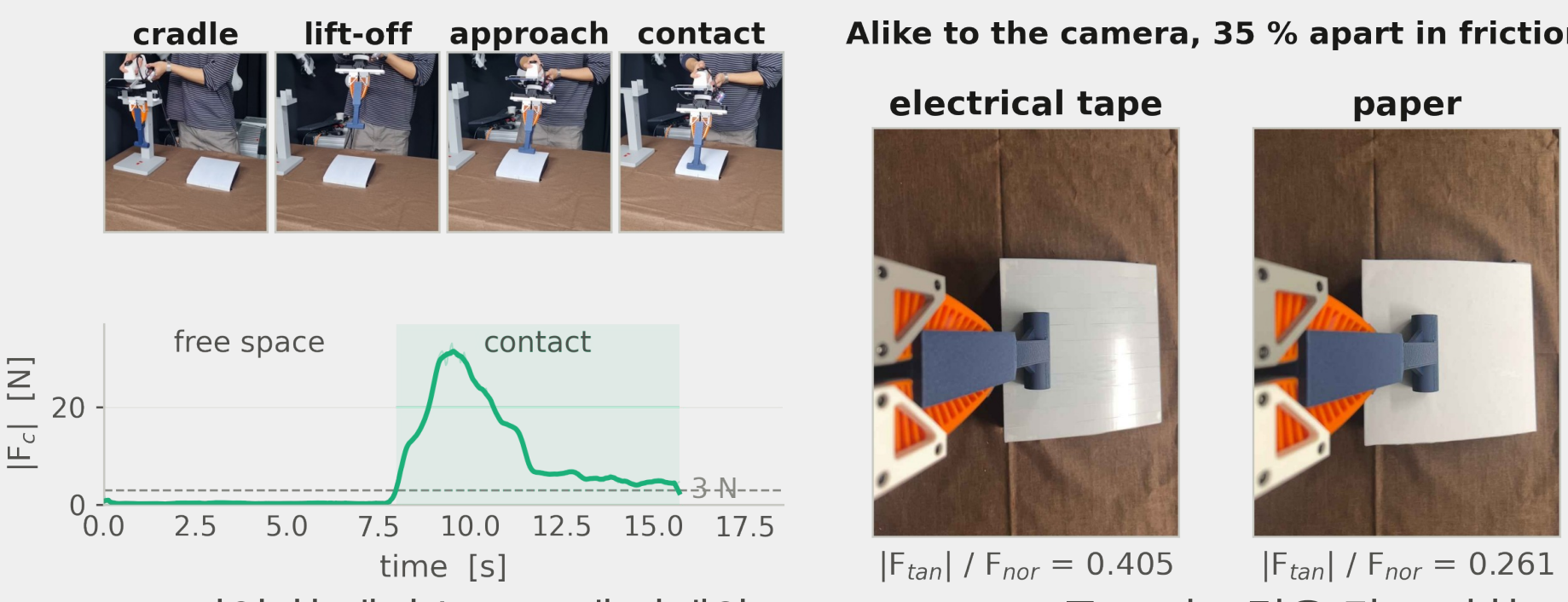
Fig. 3 시연 한 에피소드 — 네 단계와 접촉력 |F|
