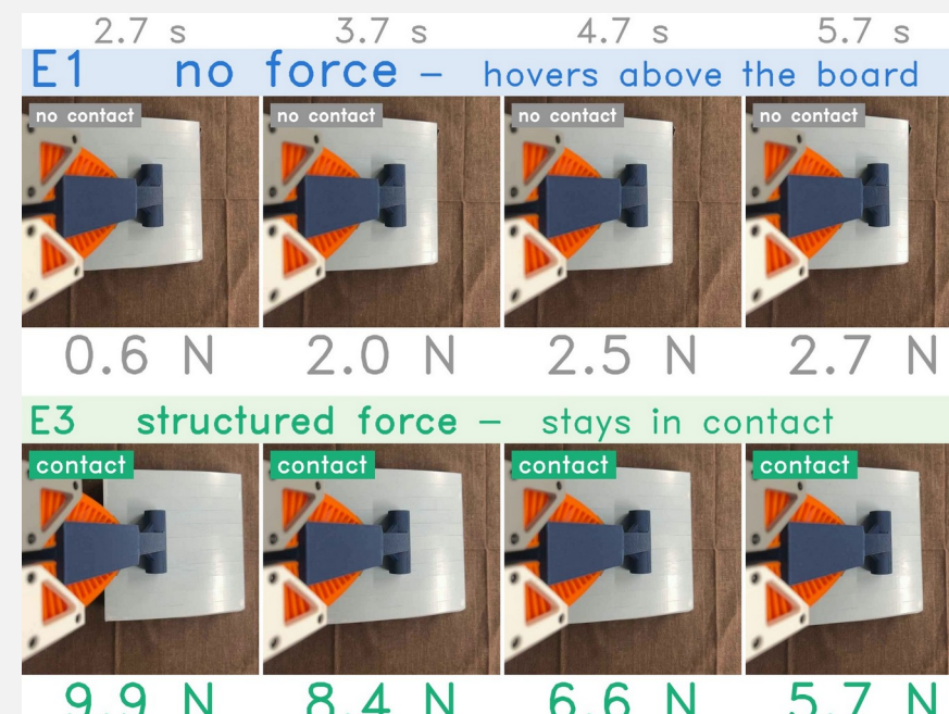
Fig. 7 FR3 페루프 — (왼쪽) 같은 그리퍼 · 톨을 단 FR3. (가운데) 한 회차, 1 초 간격. 배지 = 접촉 여부 (|F| ≥ 3 N): E1 은 판 위에 뜬 채 2 N, E3 는 눌러 미끄러진다. (오른쪽) 40 회, 점 = 회차 · 막대 = 평균
