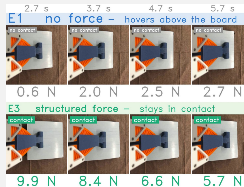
Fig. 7 FR3 페루프 — (왼쪽) 같은 그리퍼 · 톨을 단 FR3. (가운데) 한 회차, 1 초 간격. 배치 = 접촉 여부 (|F| ≥ 3 N): E1 은 판 위에 뜬 채 2 N, E3 는 눌러 미끄러진다. (오른쪽) 40 회, 점 = 회차 · 막대 = 평균. 오프라인의 차이가 실제 접촉 동작으로 이어졌고, 미학습 종이에서는 그 우세가 절반으로 준다.
