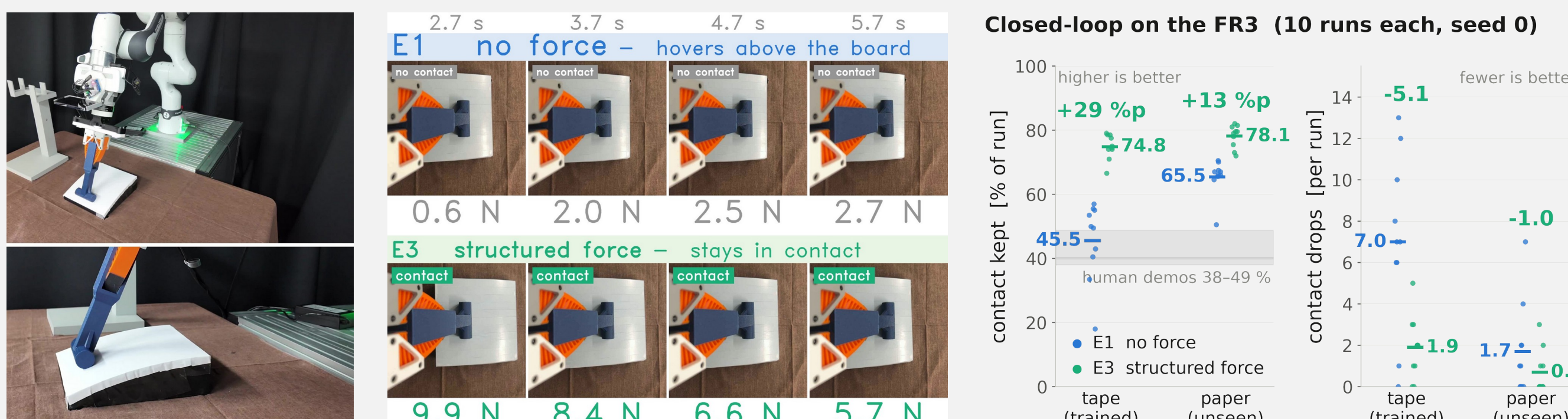
Fig. 7 FR3 페루프 — (왼쪽) 같은 그리퍼 · 툴을 단 FR3. (가운데) 한 회차, 1 초 간격. 배지 = 접촉 여부 (|F| ≥ 3 N): E1 은 판 위에 뜬 채 2 N, E3 는 눌러 미끄러진다. (오른쪽) 40 회, 점 = 회차 · 막대 = 평균
