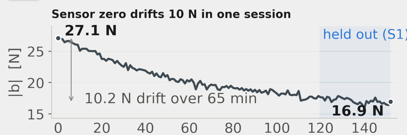
Fig. 4 센서 영점인 한 세션에 10 N 흘렀다 — 접촉력 평균 (13.6 N) 과 같은 크기다. 그래서 편향을 에피소드마다 다시 추정한다.
