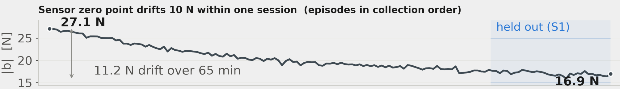
Fig. 3c 센서 영점이 한 세션에 10 N 흘렀다 — 접촉력 평균 (13.6 N) 과 같은 크기다. 그래서 편향을 에피소드마다 다시 추정한다.
