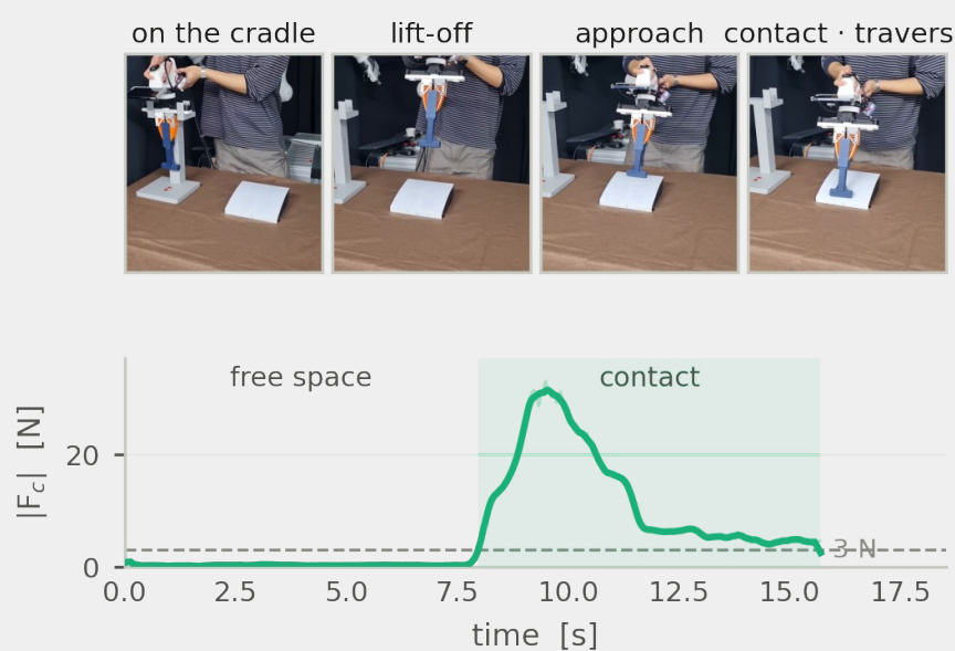
Fig. 1 과제: 바를 들어 12° 경사면에 대고 눌러 미끄러지며 추종. 아래는 한 에피소드의 접촉력 |F c | — 프레임과 힘은 서로 다른 기록이라 단계로 맞췄다.
