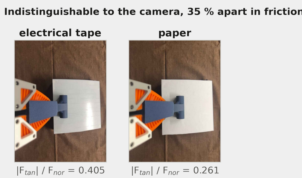
Fig. 4 두 표면 — 카메라엔 같고 마찰은 -35%
