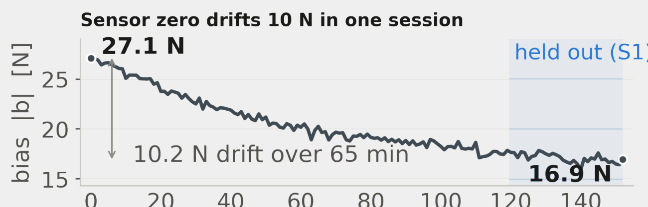
Fig. 4 센서 영점이 한 세션에 10 N 흘렀다 — 접촉력 평균 (13.6 N) 과 같은 크기
