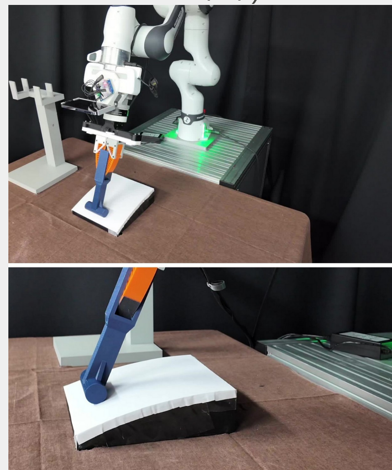
Fig. 2b 같은 그리퍼 · 같은 톨을 문 FR3
