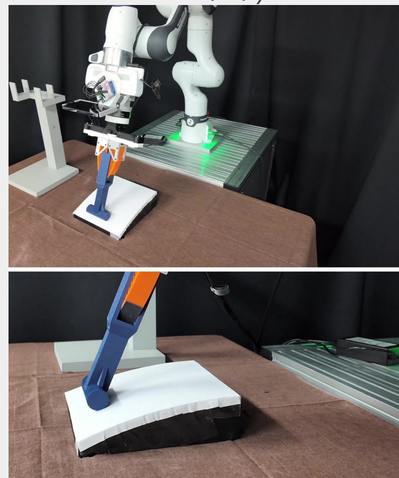
Fig. 2b 같은 그리퍼 · 같은 툴을 쓴 FR3
