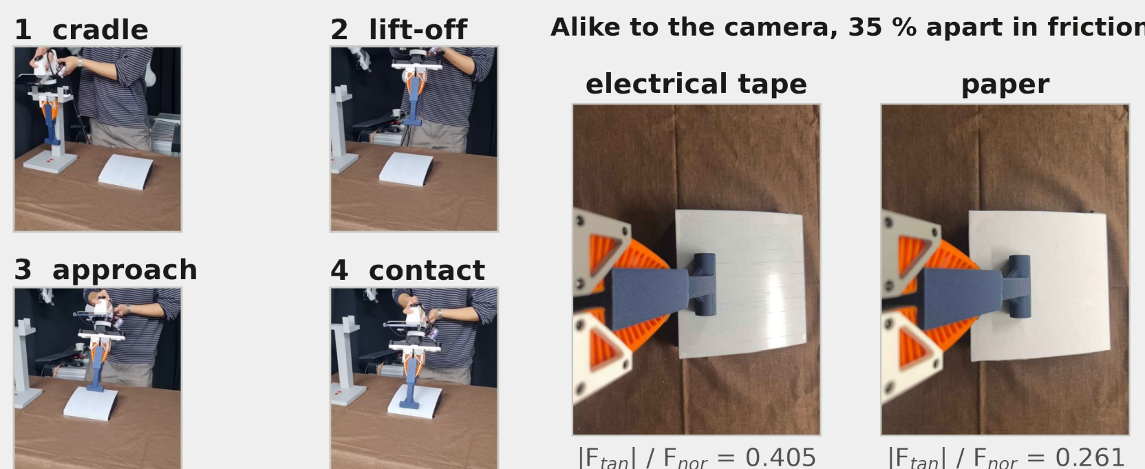
Fig. 3 시연 한 에피소드 — 들기 · 접근 · 누르며 따라가기
