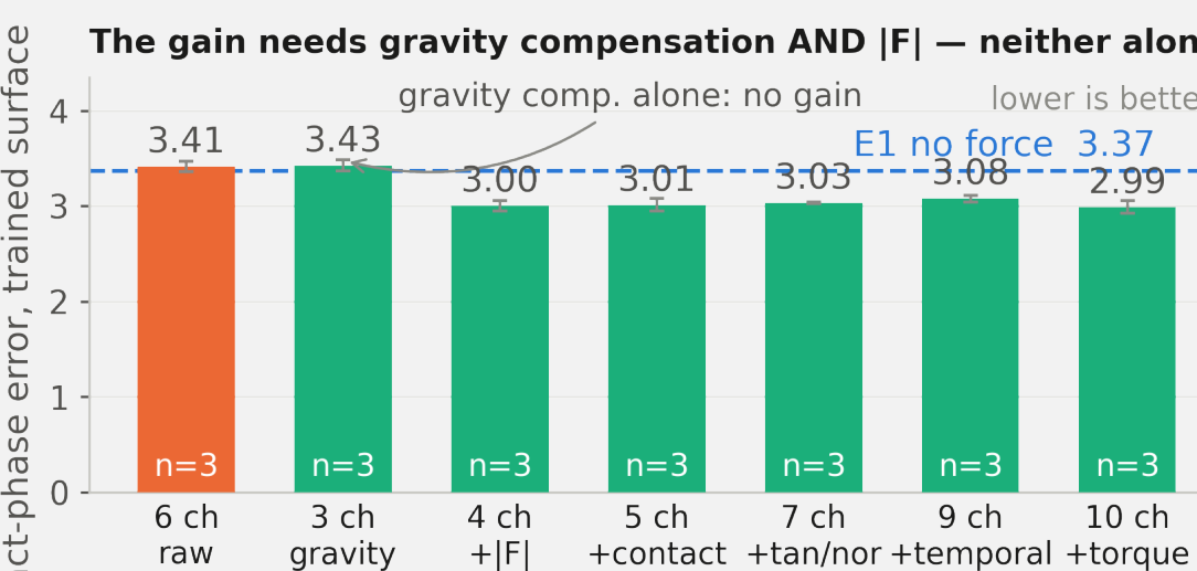
Fig. 6 이득은 중력 보상 + 힘 크기 (4 채널) 에서 나타나고, 그 뒤로는 늘지 않는다
