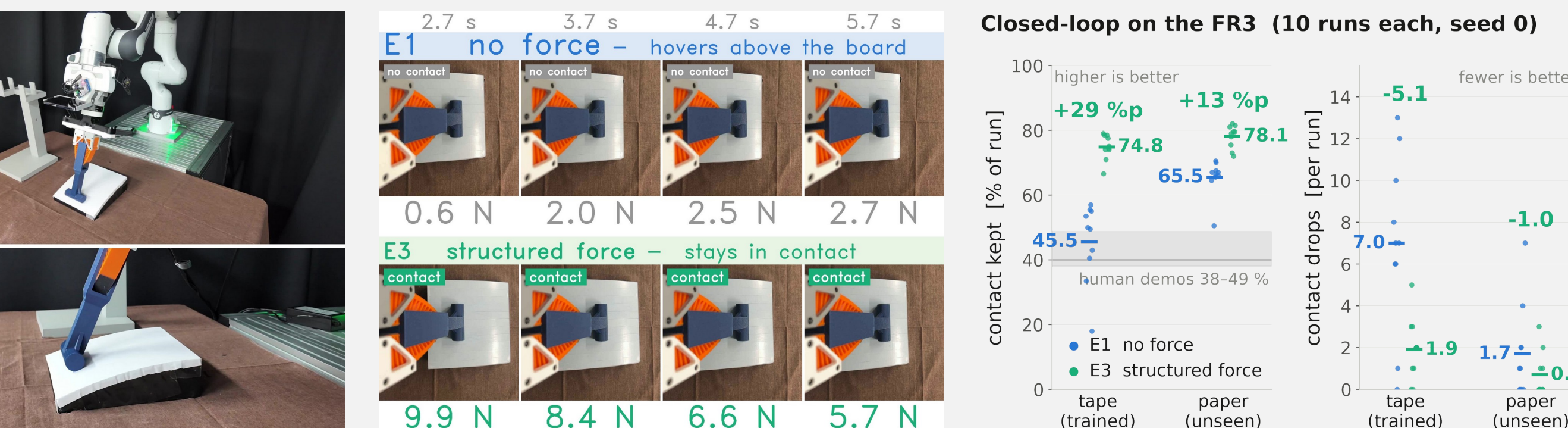
Fig. 7 FR3 페루프 — (왼쪽) 같은 그리퍼 · 툴을 단 FR3. (가운데) 한 회차, 1 초 간격. 배지 = 접촉 여부 ( |F| \geq 3 N): E1 은 판 위에 뜬 채 2 N, E3 는 눌러 미끄러진다. (오른쪽) 40 회, 점 = 회차 · 막대 = 평균
