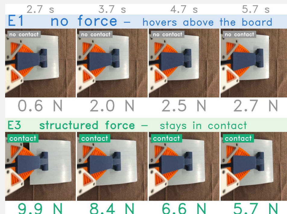
Fig. 7 FR3 페루프 — (왼쪽) 같은 그리퍼 · 톨을 단 FR3. (가운데) 한 회차, 1 초 간격. 배지 = 접촉 여부 ( |F| \geq 3 N): E1 은 판 위에 뜬 채 2 N, E3 는 눌러 미끄러진다. (오른쪽) 40 회, 점 = 회차 · 막대 = 평균
