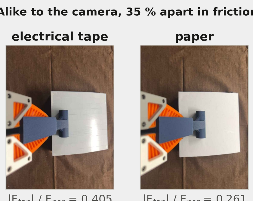
Fig. 4 두 표면: 같은 갈고 마찰 -35%
