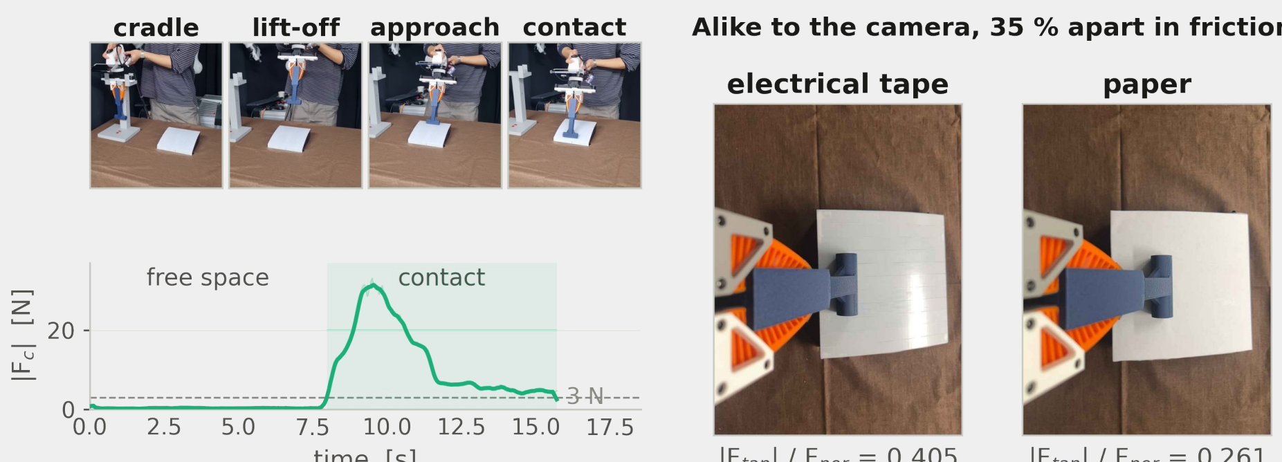
Fig. 3 시연 한 에피소드 — 네 단계와 접촉력 |F|
