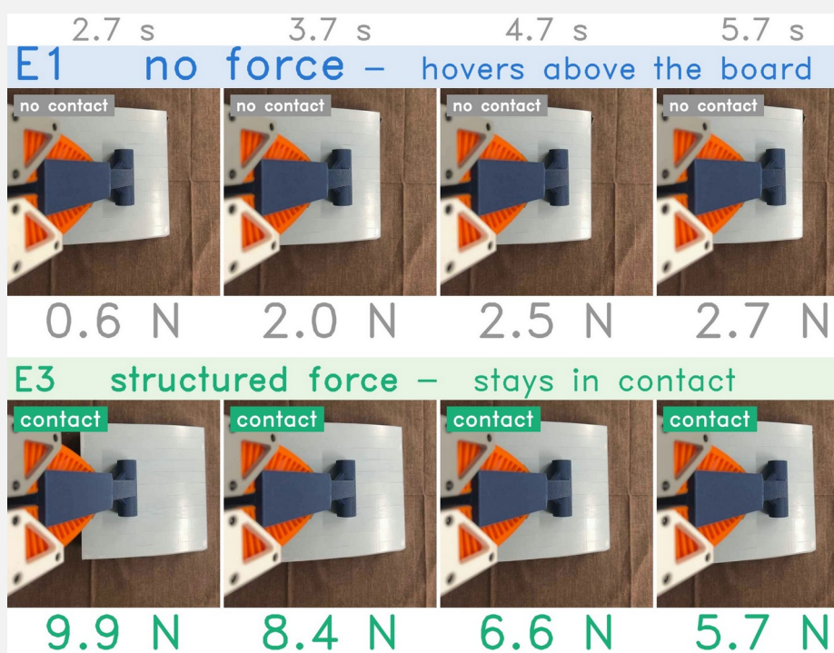
Fig. 7 FR3 페루프 — (왼쪽) 같은 그리퍼 · 톨을 단 FR3. (가운데) 한 회차, 1 초 간격. 배지 = 접촉 여부 (|F| ≥ 3 N): E1 은 판 위에 뜬 채 2 N, E3 는 눌러 미끄러진다. (오른쪽) 40 회, 점 = 회차 · 막대 = 평균
