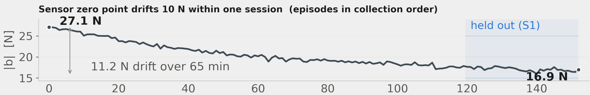
Fig. 3c 센서 영점이 한 세션에 10 N 흘렀다 — 접촉력 평균 (13.6 N) 과 같은 크기다. 그래서 편향을 에피소드마다 다시 추정한다.
