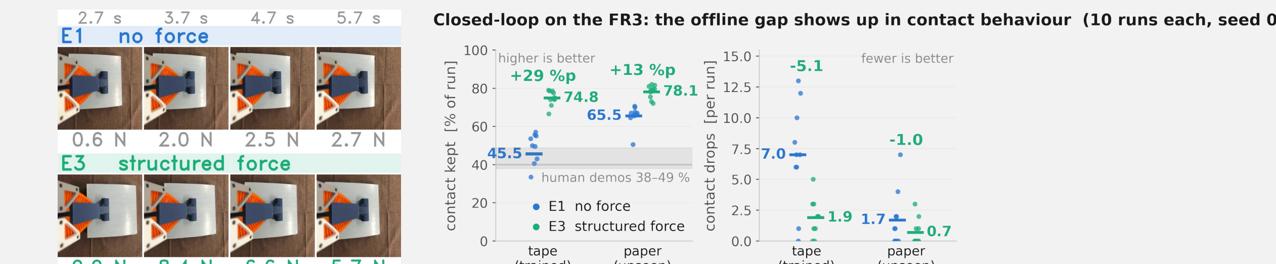
Fig. 7 (왼쪽) 한 회차를 1 초 간격으로 — 힘 없음 (E1) 은 판을 놓친 채 2 N 대에 머물고, 구조화 (E3) 는 눌러 미끄러진다 (접촉 기준 3 N). (오른쪽) FR3 페루프 40 회, 점 = 회차 · 막대 = 평균.
