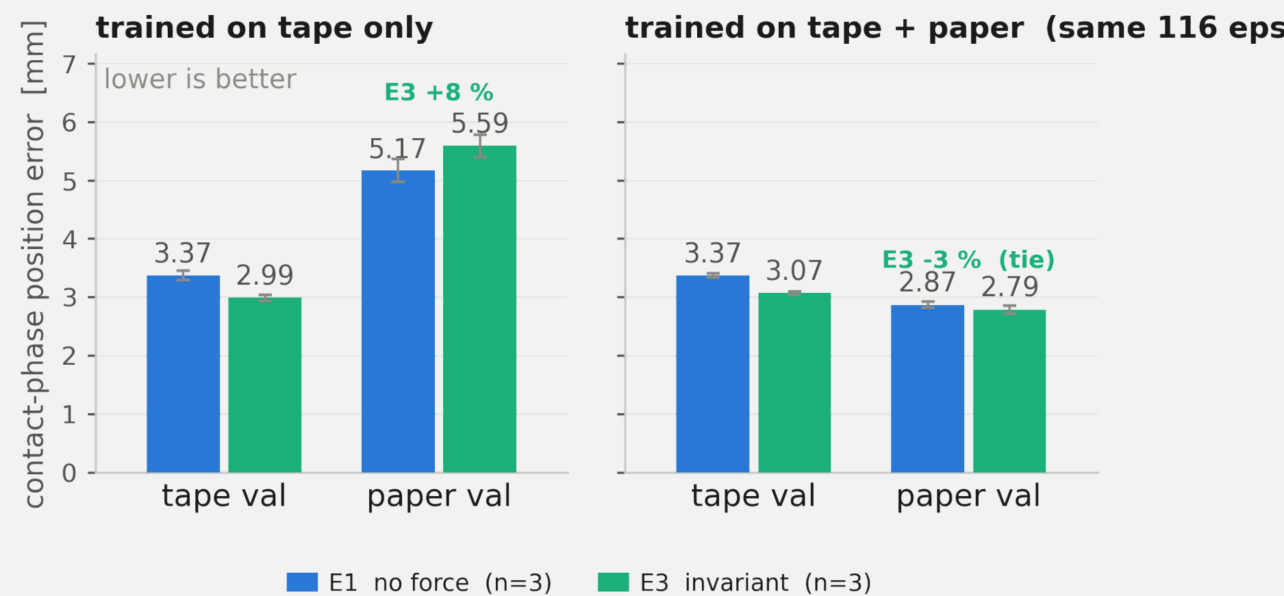
Fig. 6 단일 표면 학습 (왼쪽) 과 혼합 학습 (오른쪽) 에서 E1 vs E3. 종이 값은 겹중 34 개 기준이라 표 (150 개 전체) 와 다르다.
