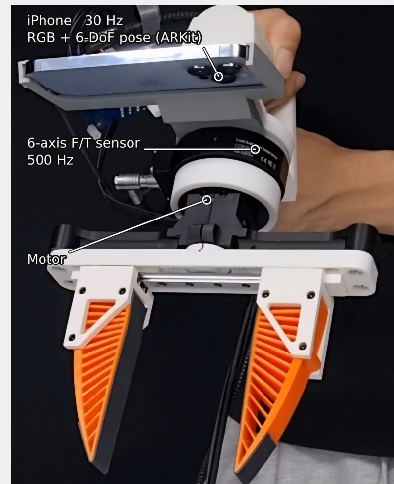
Fig. 2a 제작한 수집 장치 (손목 F/T 추가)
