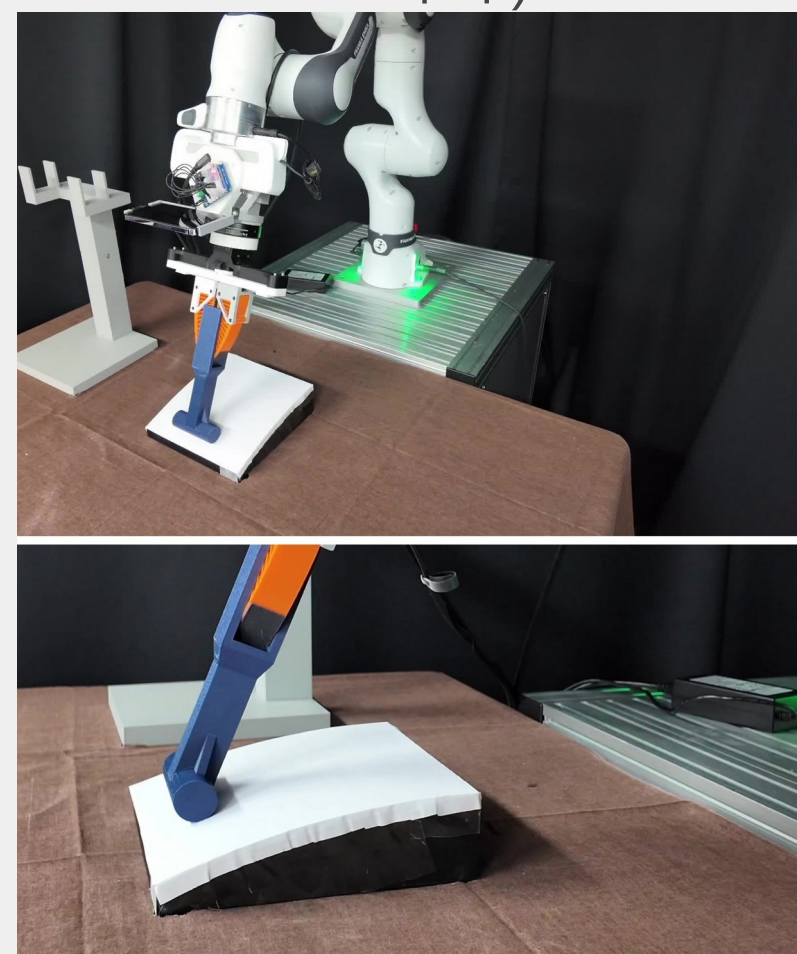
Fig. 2b 같은 그리퍼 · 같은 툴을 문 FR3 — 09-18 실기 장면
