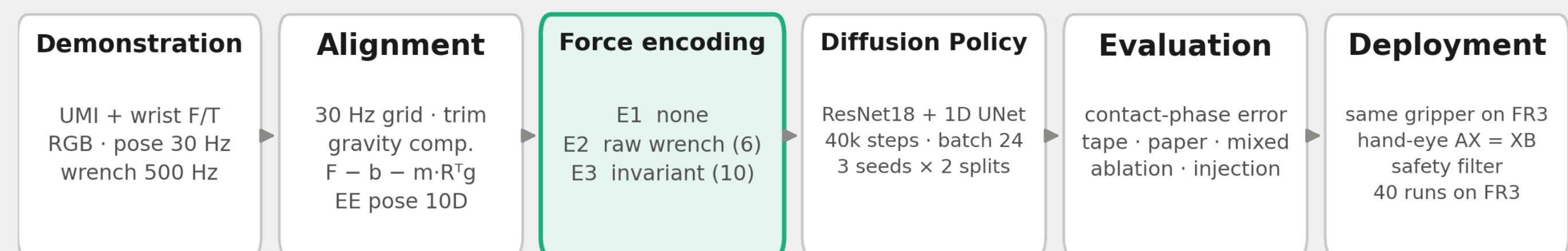
Fig. 2 파이프라인 — 세 정책은 힘 표현 단계만 다르다
