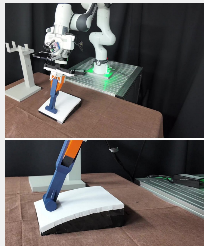
Fig. 3b 같은 그리퍼 · 같은 툴을 문 FR3 — 09-18 실기 장면
