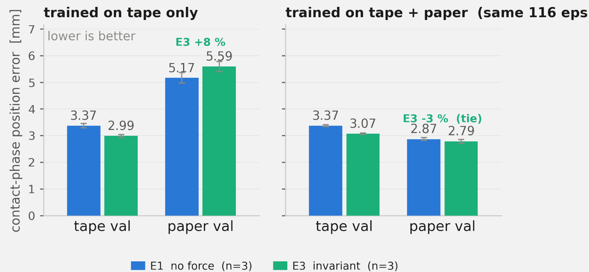
Fig. 5 단일 표면 학습 (왼쪽) 과 혼합 학습 (오른쪽) 에서 E1 vs E3
