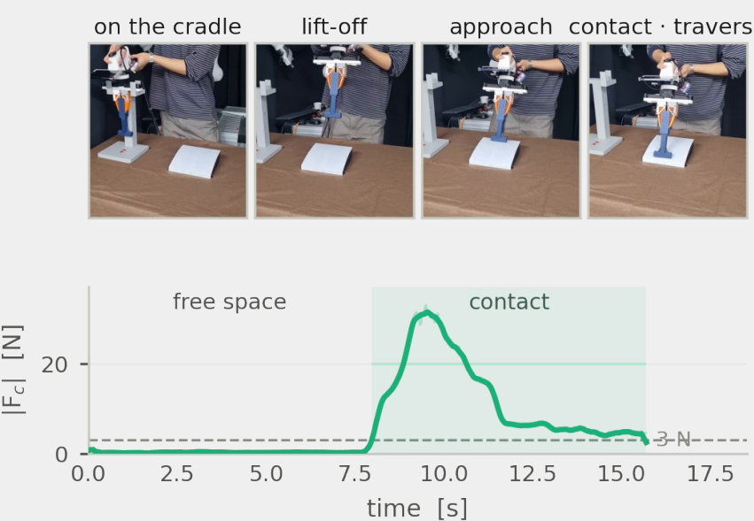
Fig. 1 과제: 바를 들어 12° 경사면에 대고 눌러 미끄러지며 추종. 아래는 한 에피소드의 접촉력 |F| — 프레임과 힘은 서로 다른 기록이라 단계로 맞췄다.
