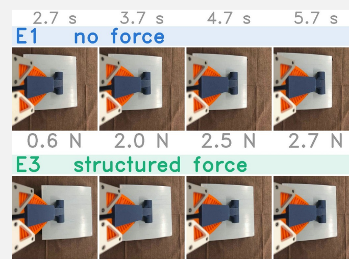
Fig. 7 (왼쪽) 한 회차를 1 초 간격으로 — 힘 없음 (E1) 은 판을 놓친 채 2 N 대에 머물고, 구조화 (E3) 는 눌러 미끄러진다 (접촉 기준 3 N). (오른쪽) FR3 페루프 40 회, 점 = 회차 · 막대 = 평균.
