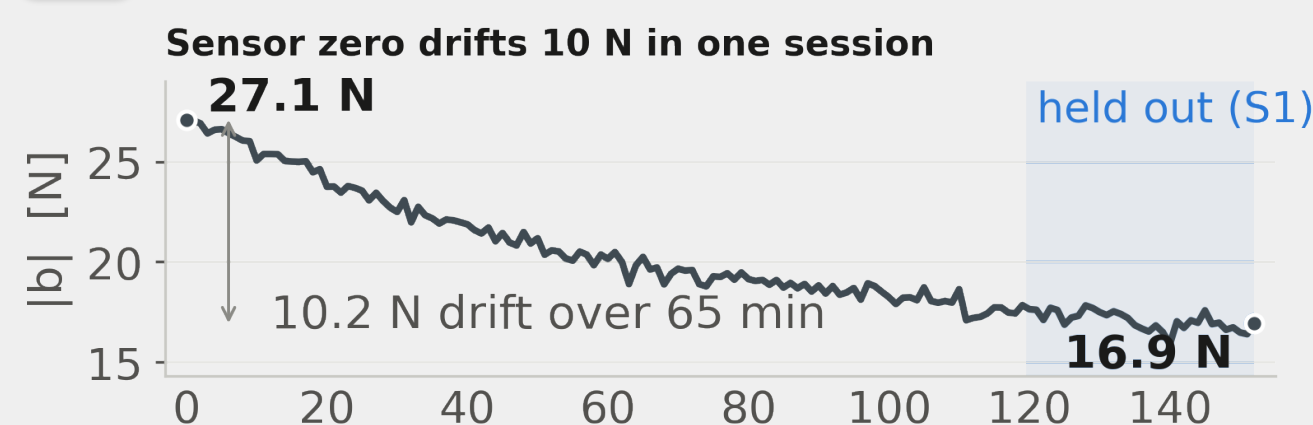
Fig. 4 센서 영점이 한 세션에 10 N 흘렀다 — 접촉력 평균 (13.6 N) 과 같은 크기다. 그래서 편향을 에피소드마다 다시 추정한다.
