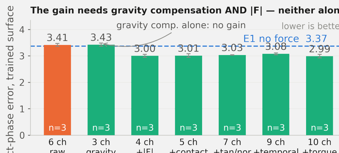
Fig. 7 이득은 중력 보상 + 힘 크기 (4 채널) 에서 나타나고, 그 뒤로는 늘지 않는다
