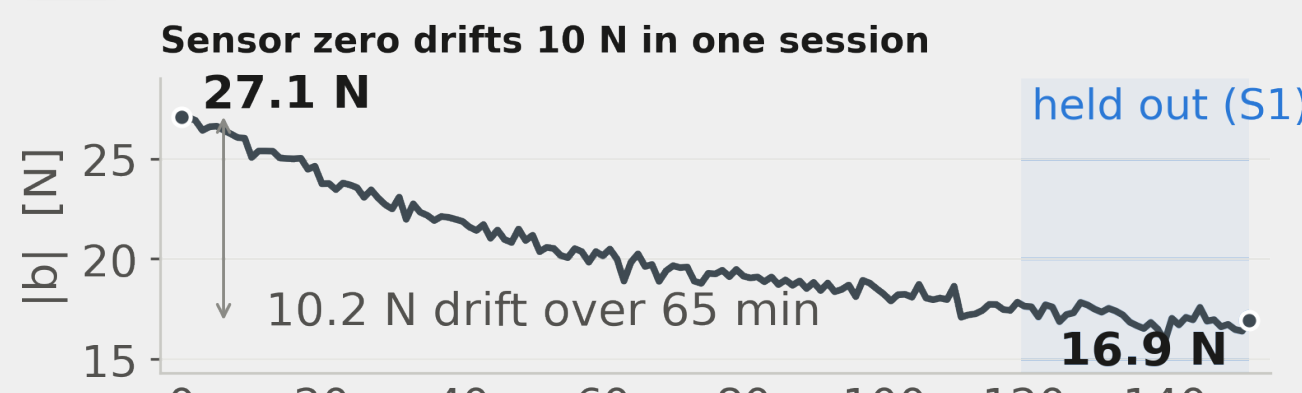
Fig. 5 센서 영점이 한 세션에 10 N 흘렀다 — 접촉력 평균 (13.6 N) 과 같은 크기다. 그래서 편향을 에피소드마다 다시 추정한다.
