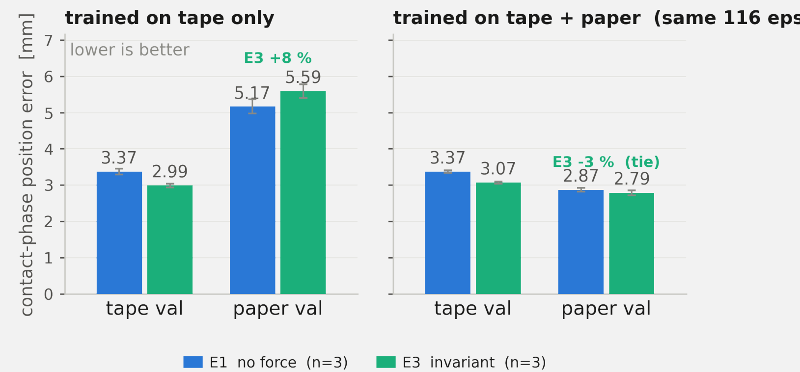
Fig. 6 단일 표면 학습 (왼쪽) 과 혼합 학습 (오른쪽) 에서 E1 vs E3. 종이 값은 검증 34 개 기준이라 표 (150 개 전체) 와 다르다.
