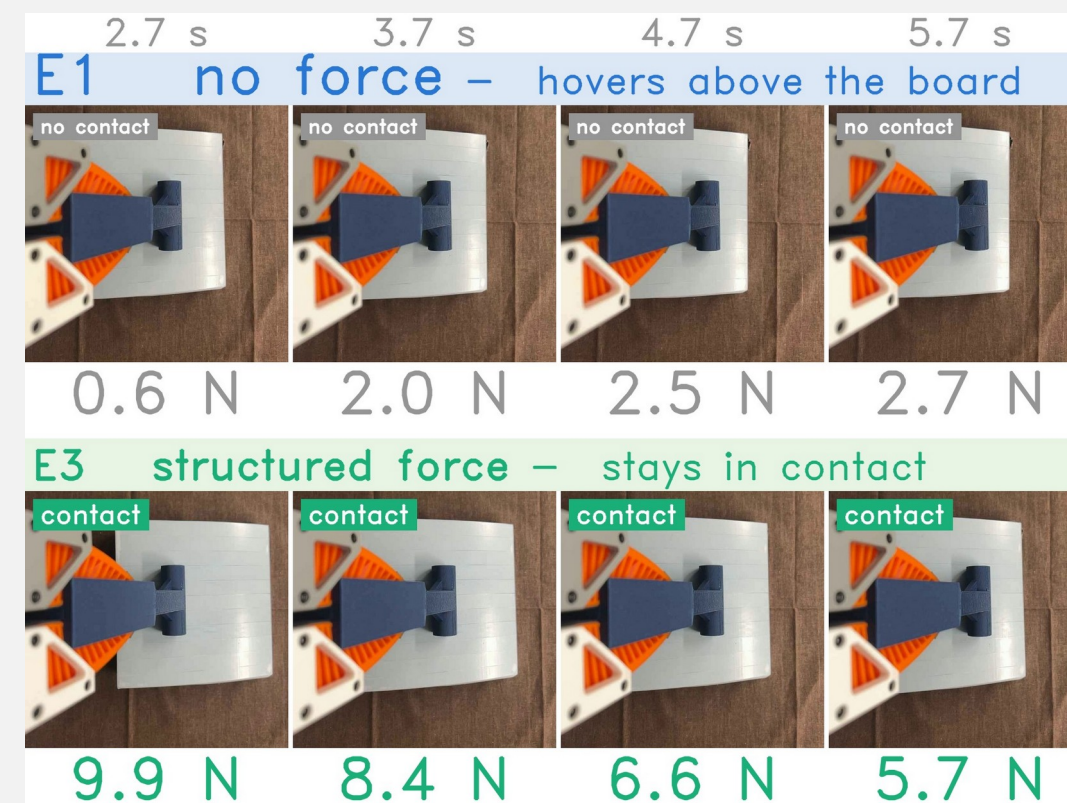
Fig. 8 FR3 페루프 — (왼쪽) 한 회차, 1 초 간격. 배지 = 접촉 여부 ( |F| \geq 3 N): E1 은 판 위에 뜬 채 2 N, E3 는 눌러 미끄러진다. (오른쪽) 40 회, 점 = 회차 · 막대 = 평균
