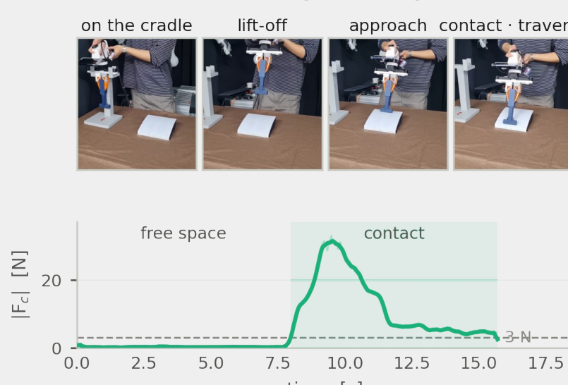
Fig. 3 시연 한 에피소드 — 네 단계와 접촉력 |F|
