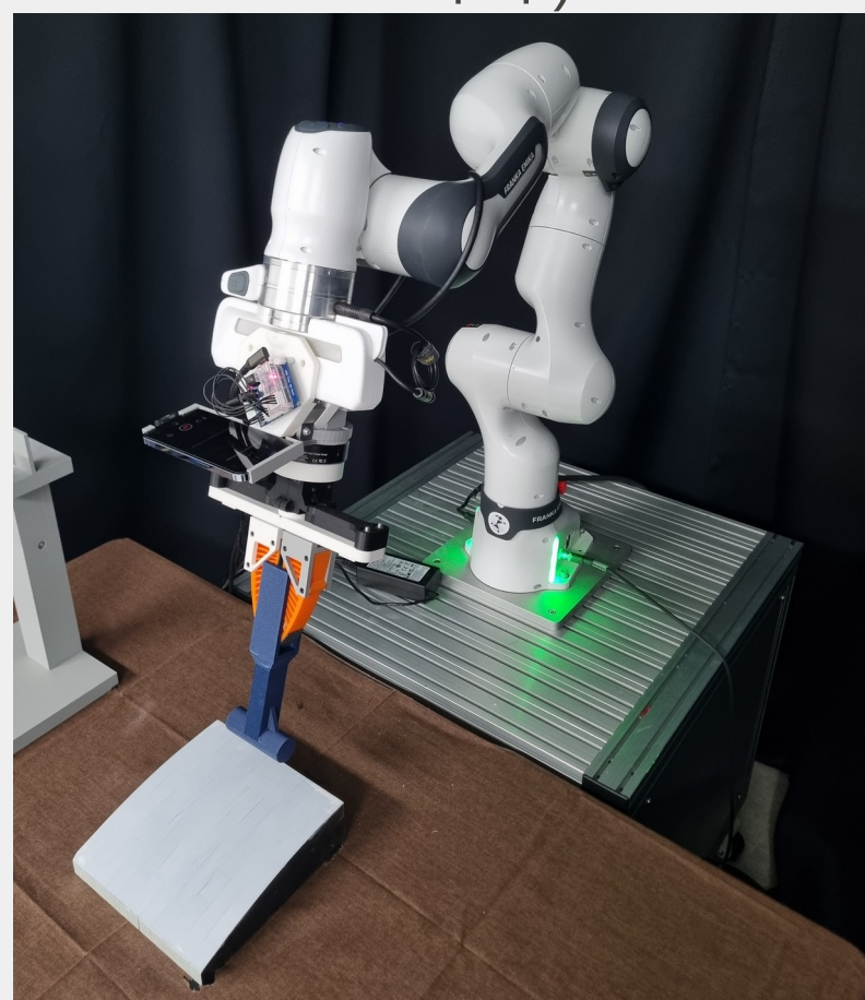
Fig. 2b 같은 그리퍼 · 같은 툴을 문 FR3 — 09-18 실기 장면
