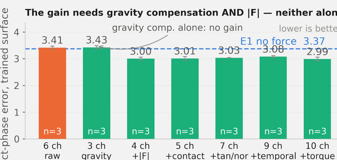
Fig. 7 이득은 중력 보상 + 힘 크기 (4 채널) 에서 나타나고, 그 뒤로는 늘지 않는다
