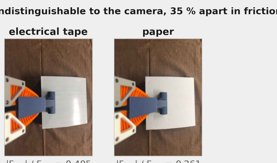
Fig. 4 두 표면: 같은 같고 마찰은 ~35%
