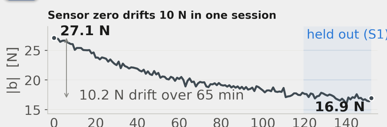
Fig. 5 센서 영점이 한 세션에 10 N 흘렀다 — 접촉력 평균 (13.6 N) 과 같은 크기다. 그래서 편향을 에피소드마다 다시 추정한다.
