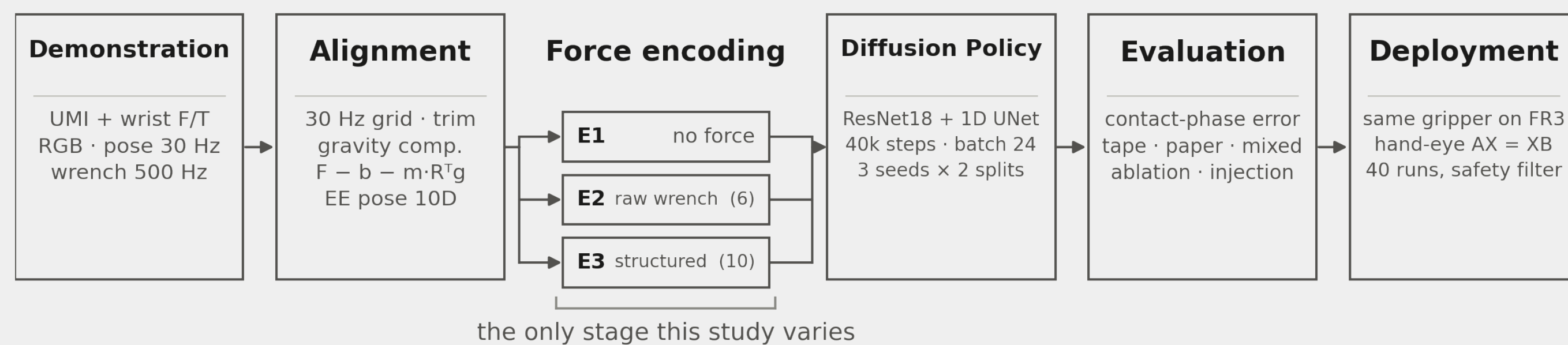
Fig. 1 파이프라인 — 세 정책은 힘 표현 단계만 다르다
