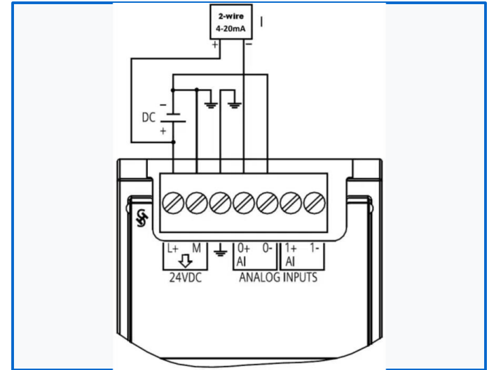
Integração: Sinais de campo (4-20mA) processados pelo CLP e enviados ao Supervisório
