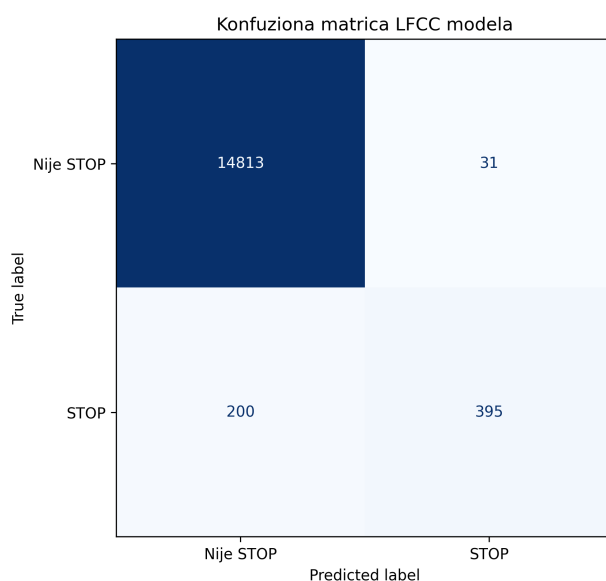
Slika 7: Konfuzionna matrica LFCC modela
