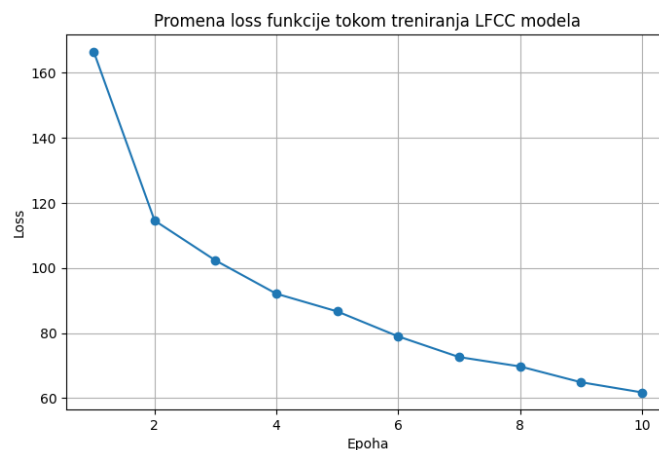
Slika 6: Promena vrednosti funkcije gubitka tokom treniranja LFCC modela
