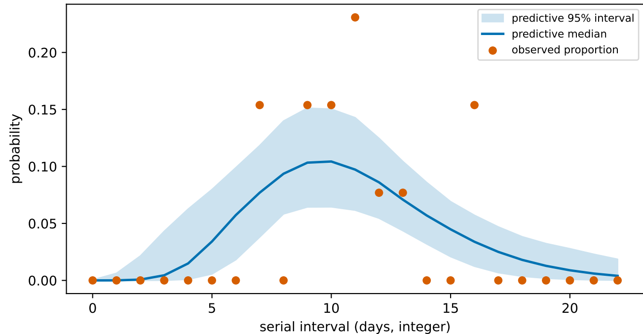
Posterior predictive check - high only
